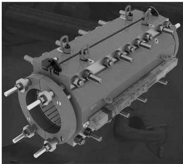
Рисунок А.1 — Общий вид стальной ремонтной муфты
