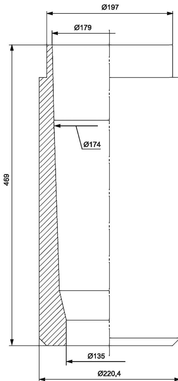
Рисунок 3 — Прошивная матрица
