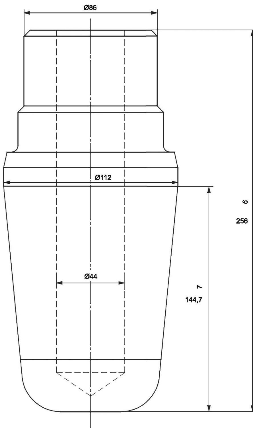
Рисунок 2 — Головка прошивного пуансона
