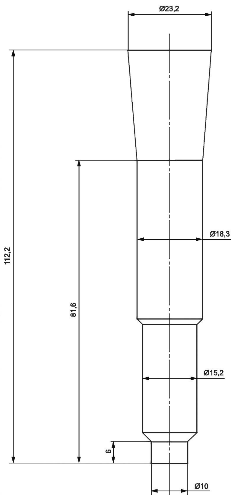
Рисунок 1 — Пуансон холодного выдавливания
