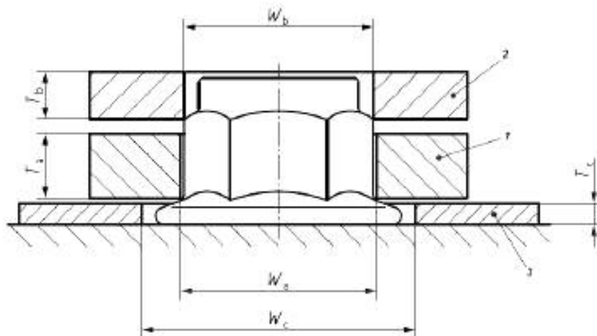
1 — Калибр А; 2 — Калибр В; 3 — Калибр С
