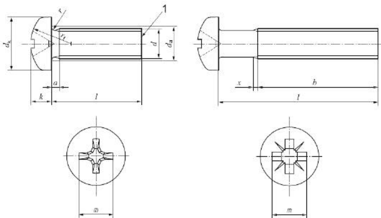
а) Крестообразный шлиц типа Н
