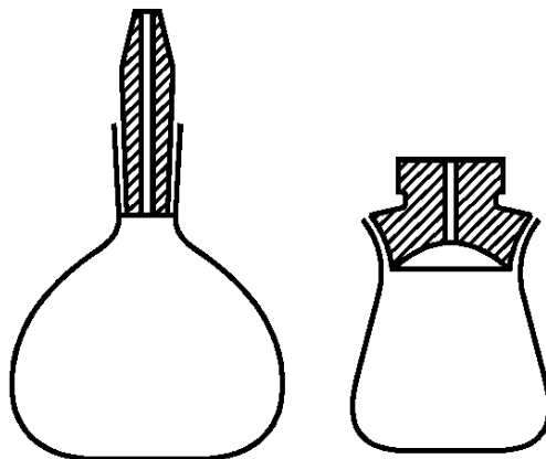
Рисунок 1 — Пикнометры
