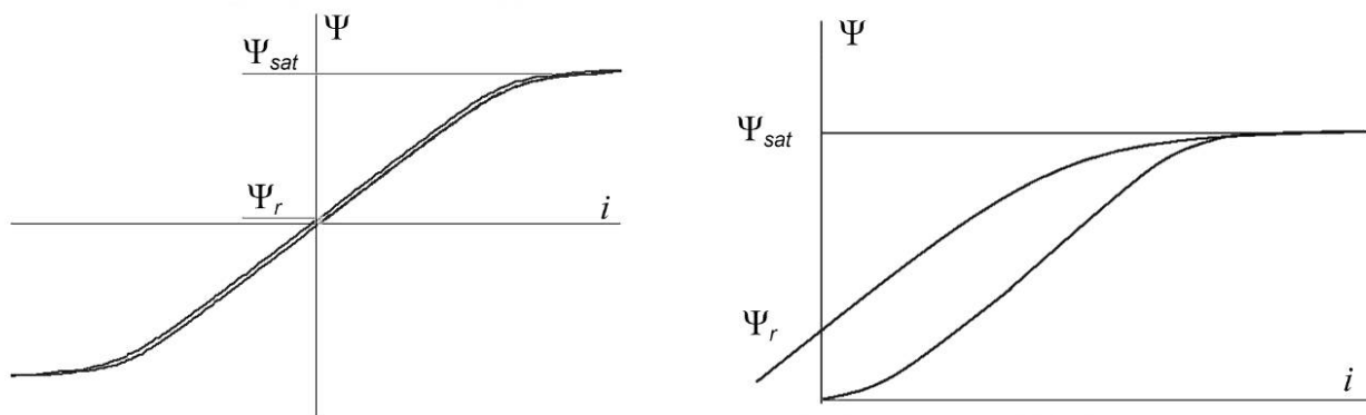
а) Пример определения остаточной намагниченности при использовании источника синусоидального напряжения
