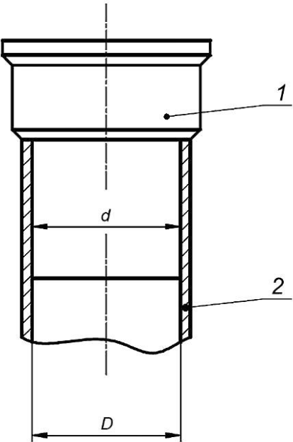
1 — окуляр; 2 — тубус
