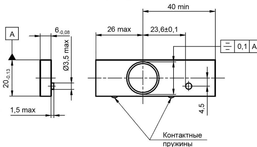
Рисунок 6 — Присоединительные размеры тубусных вставок
