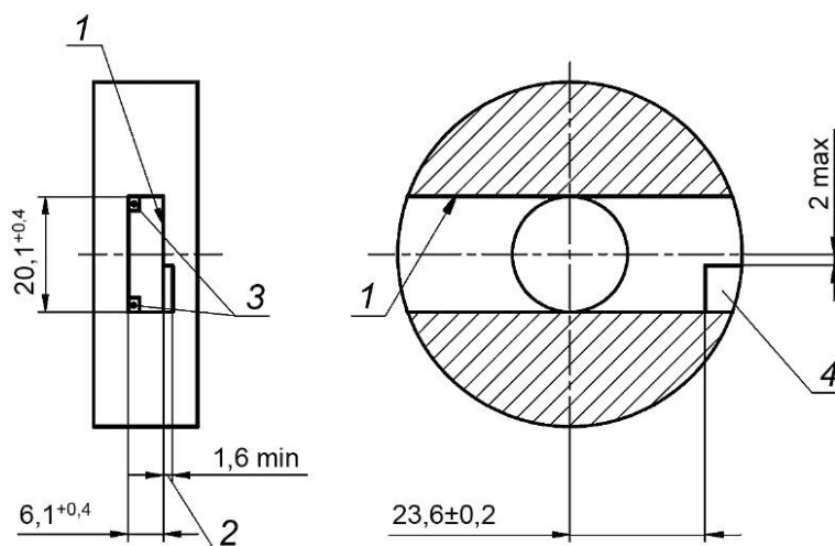
Рисунок 6 — Присоединительные размеры тубусных вставок
