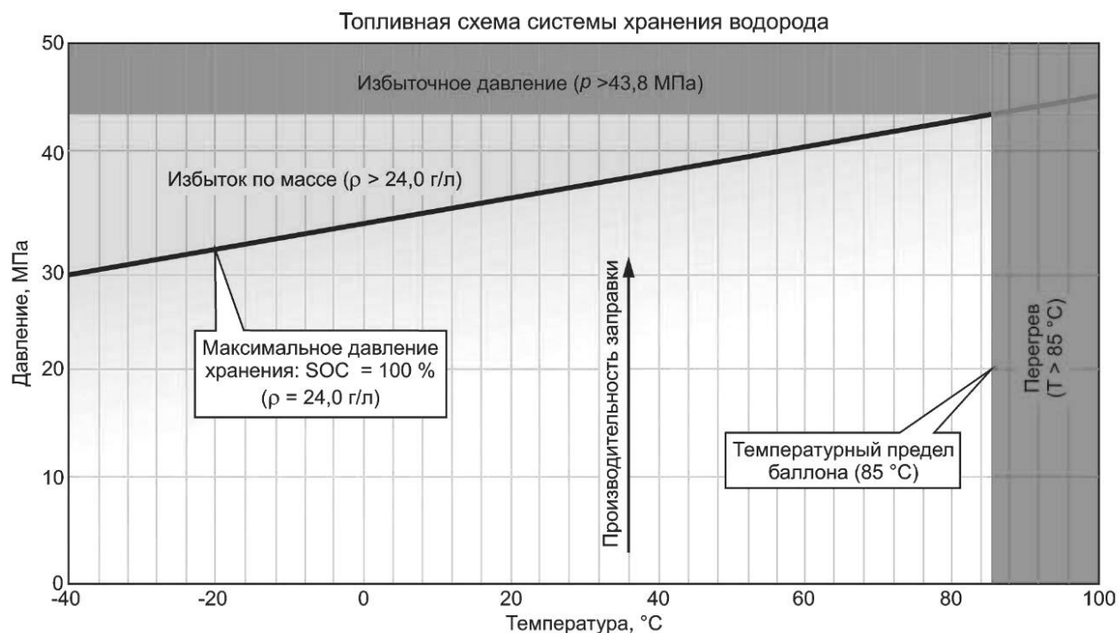
Рисунок 1 — Нормальные граничные условия Н35
