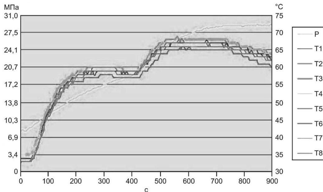
Рисунок 2 — Пример показаний датчиков давления и температуры при заправке
