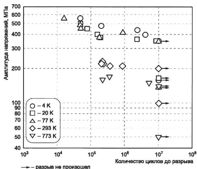
Рисунок В.4 — Данные по усталостной долговечности нержавеющей стали типа 304L, испытанной в средах жидкого гелия (4 К), жидкого водорода (20 К), жидкого азота (77 К) и температуры окружающей среды (293 К и 773 К)
