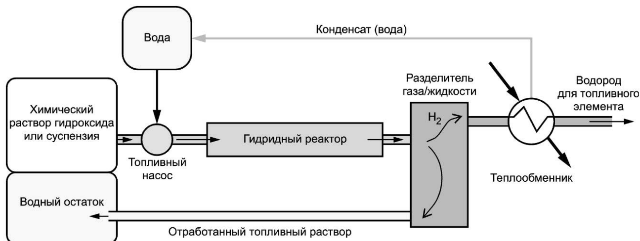
Рисунок 2 — Упрощенная схема системы хранения водорода на основе гидридов с химическим методом извлечения водорода
