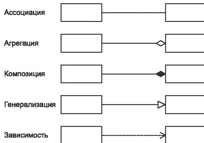
Рисунок 1 — Символика UML
