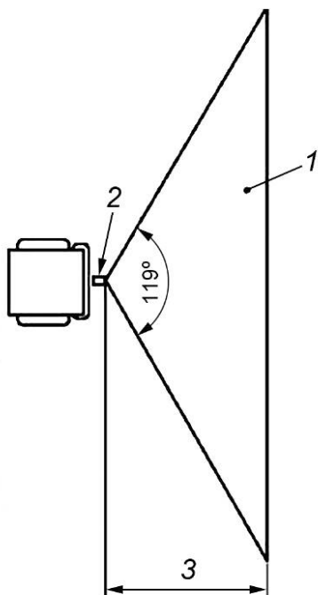
1 — зарегистрированные угол и сектор; 2 — камера; 3 — дальность в метрах
