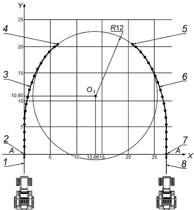
Рисунок А.2 — Траектории движения РВАМТА с рулевым управлением в аварийном состоянии (время движения 8 с)
