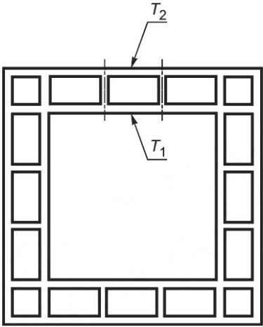
T_1 , T_2 — внутренняя температура поверхности полости трубы
