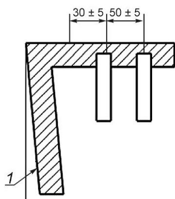
а) Продольное сечение шаблона
