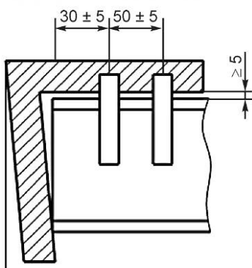
а) Продольное сечение шаблона
