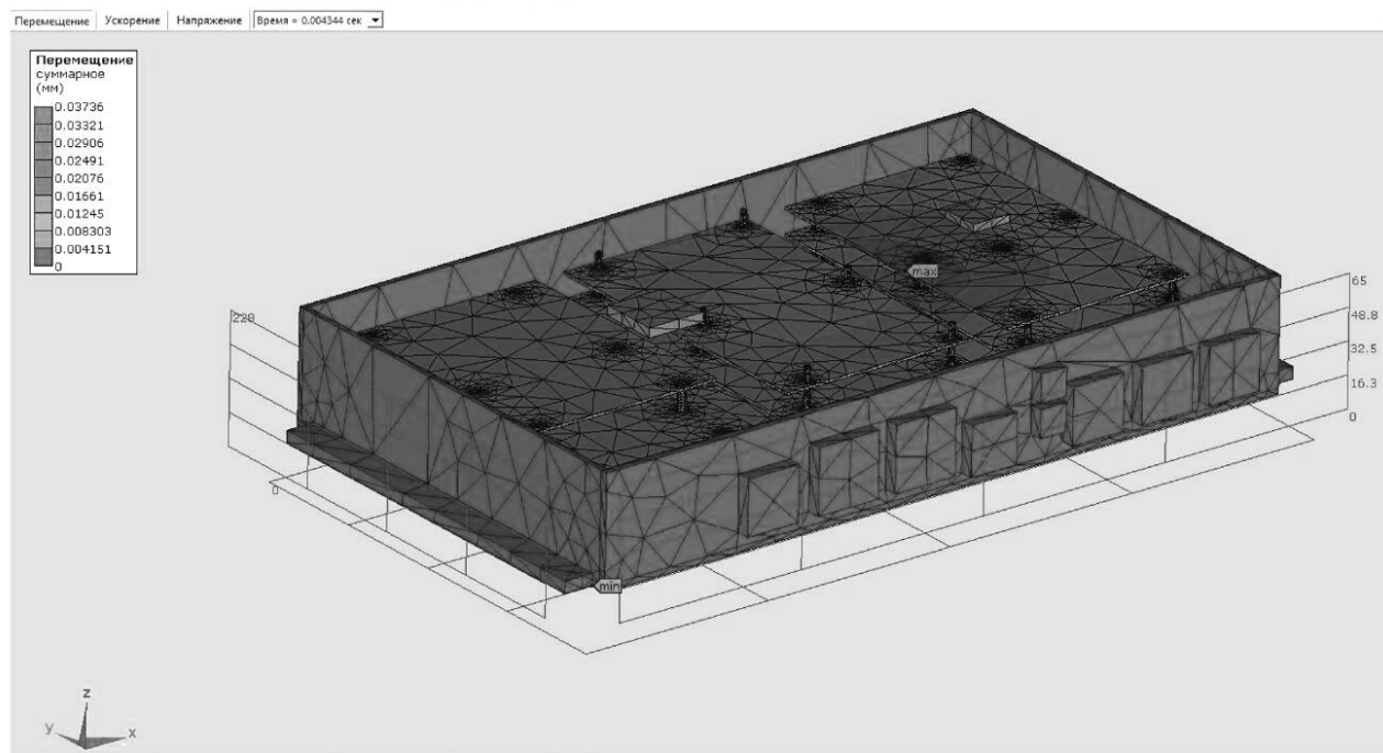
Рисунок А.6 — Суммарные перемещения во всех точках конструкции блока ЭА при воздействии одиночного механического удара в заданный момент времени
