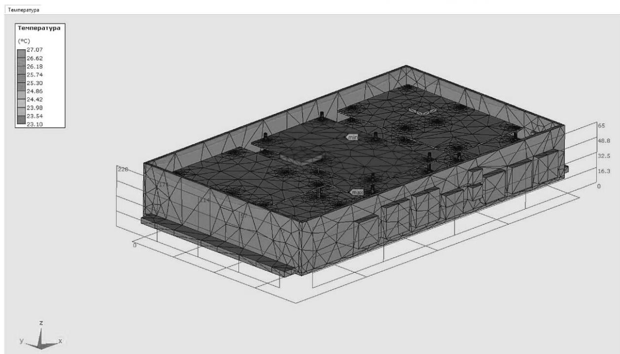
Рисунок А.11 — Температуры во всех точках конструкции блока ЭА
