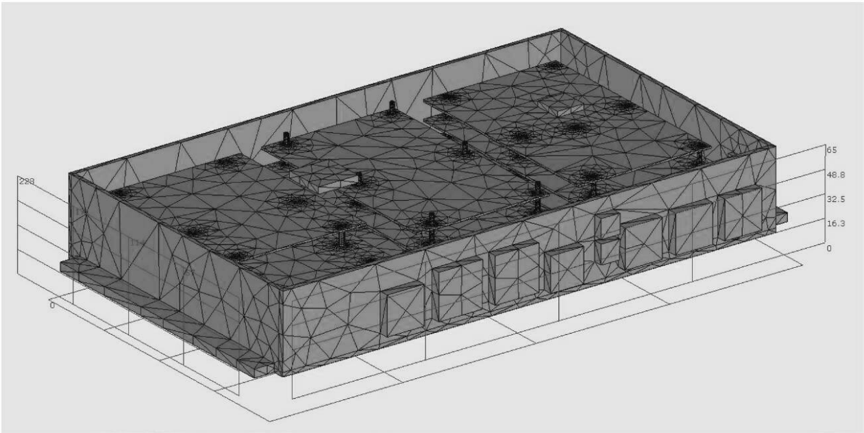
Рисунок А.5 — Автоматическое разбиение на конечные элементы
