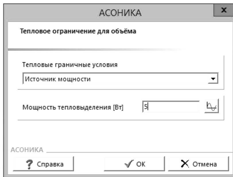
Рисунок А.10 — Задание источника постоянной мощности
