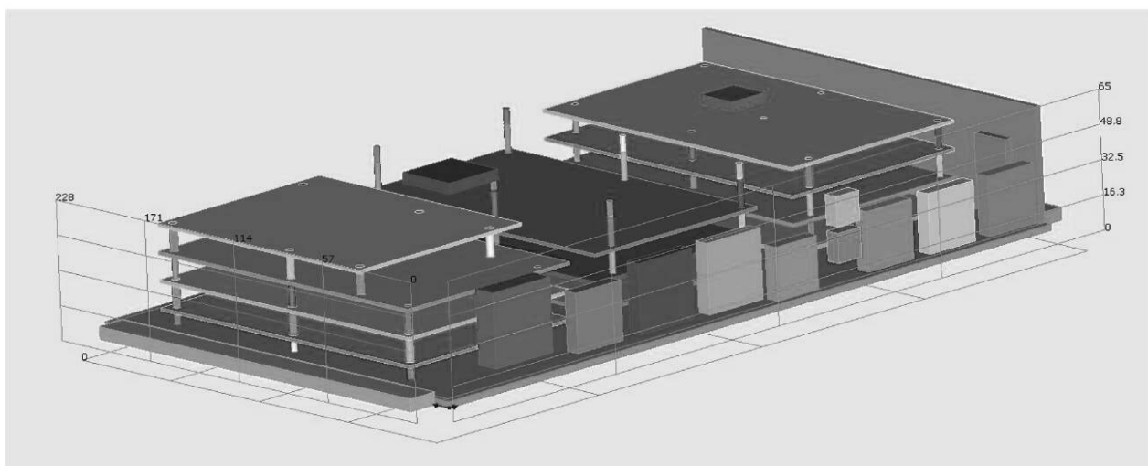
Рисунок А.4 — Конструкция блока ЭА, импортированная из CAD-системы в подсистему АСОНИКА-М-3D
