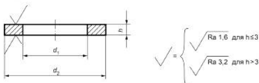
Рисунок 1 — Размеры
