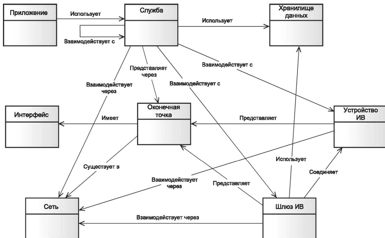
Рисунок 7 — Службы, сети, устройства и шлюзы ИВ
