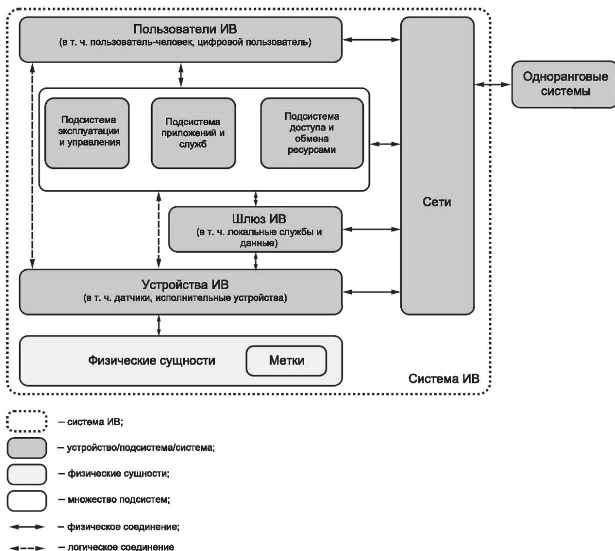
Рисунок 11 — Типовая модель на основе сущностей
