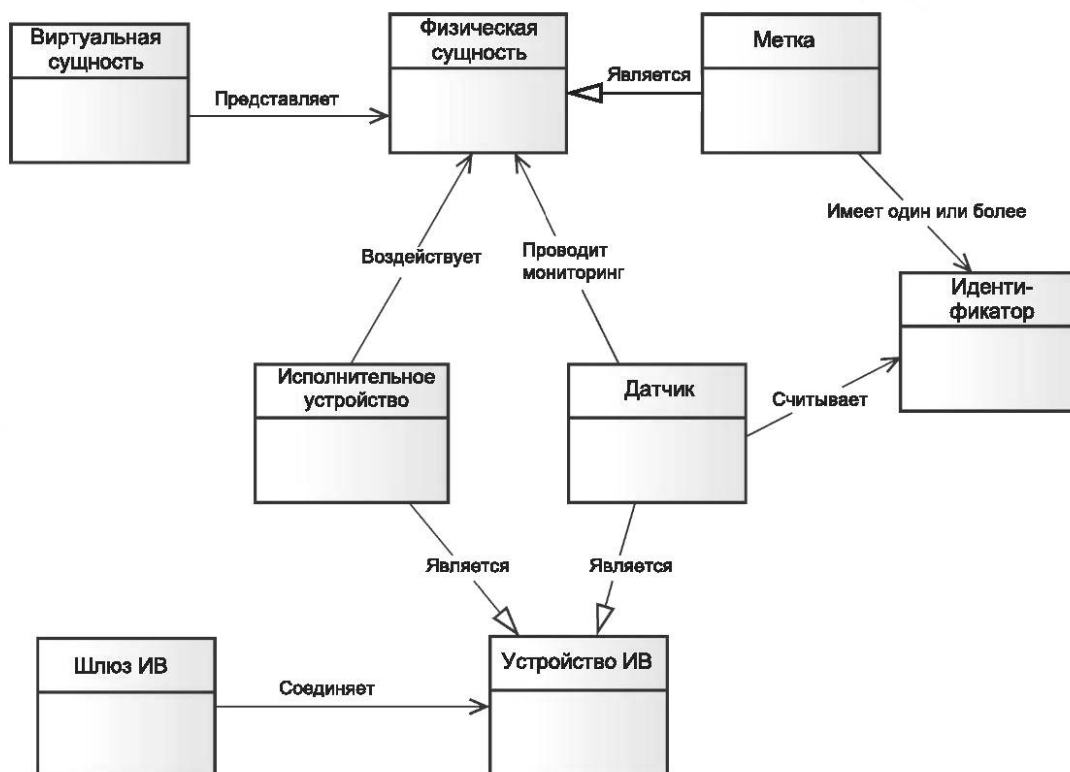
Рисунок 9 — Понятия виртуальной сущности, физической сущности и устройства ИВ
