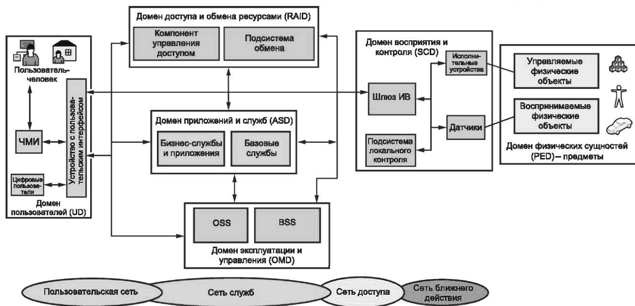
Рисунок 16 — Представление развертывания типовой архитектуры ИВ
