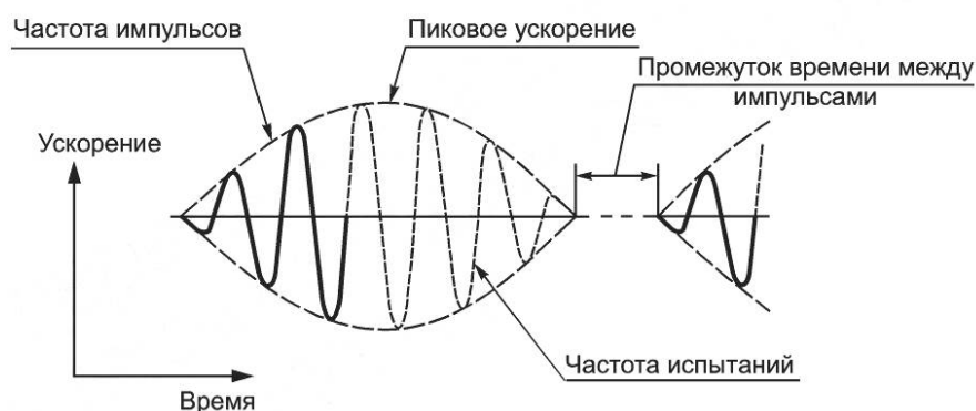
Рисунок 1 — Синусоидальные импульсы
