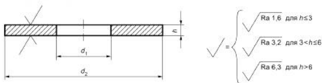
Рисунок 1 — Размеры
