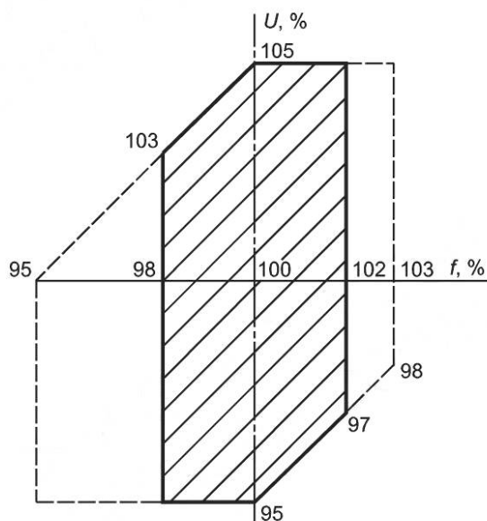
Рисунок 1 — Диапазоны допустимых изменений напряжения и частоты
