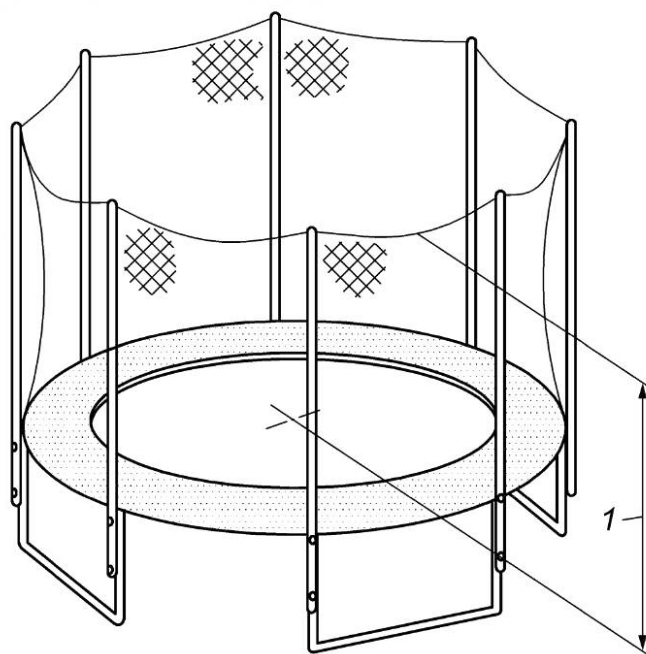
Рисунок 1 — Высота защитной сетки
