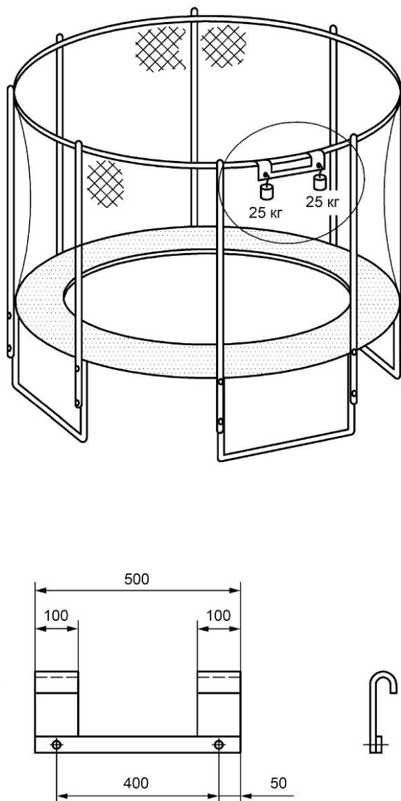
Рисунок 8 — Пример держателя для грузов
