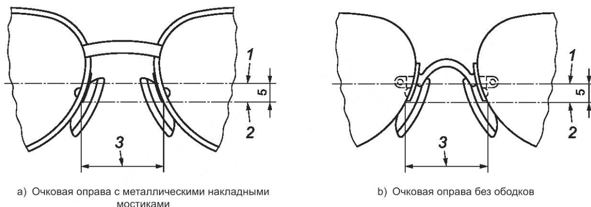
Рисунок 6 — Ширина носовой перемычки
