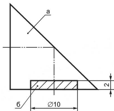
Рисунок 17 — Объем контроля
