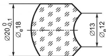
Рисунок 13 — Контролируемая область
