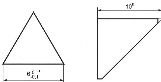
Рисунок 30 — Линейные размеры для призм
