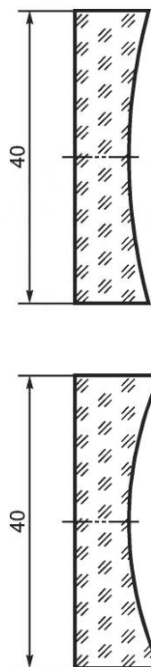
Рисунок 6 — Торическая линза
