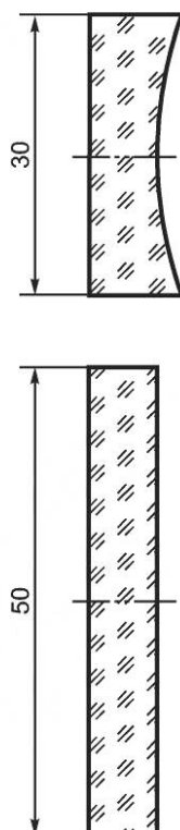
Рисунок 5 — Цилиндрическая линза
