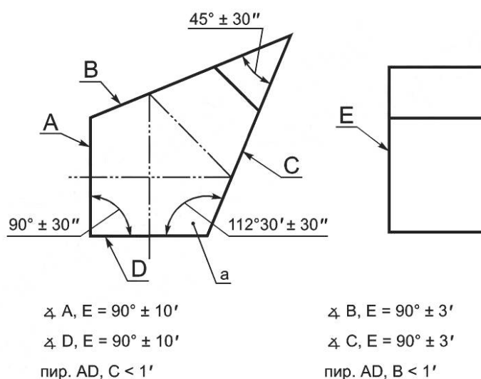
Рисунок 31 — Углы с допусками
