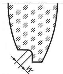
Рисунок 28 — Обозначения ширины скругления внутренней кромки
