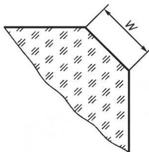
Рисунок 26 — Ширина защитной фаски W
