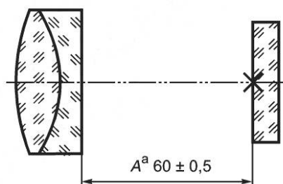
Рисунок 37 — Оптическая система с регулируемым воздушным промежутком
