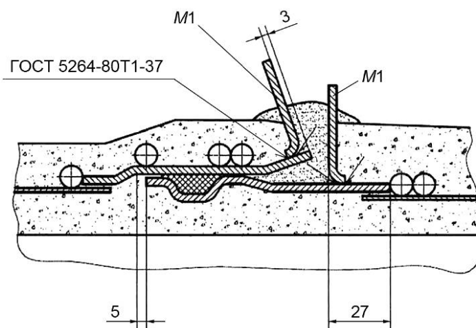
Рисунок Б.6 — Схема размещения (приварки) закладных деталей ПЭ к раструбу и втулке стыкуемых труб
