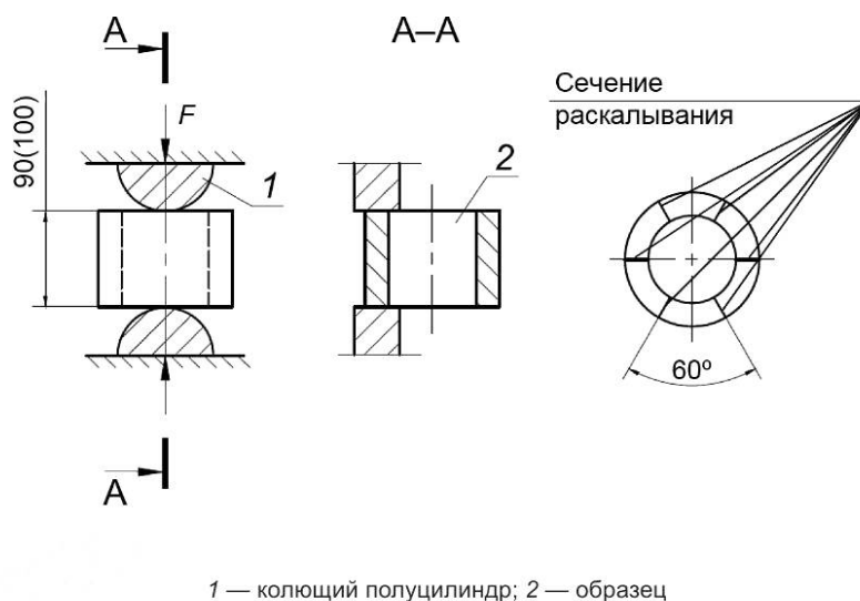
Рисунок В.1 — Схема испытания бетонных образцов
