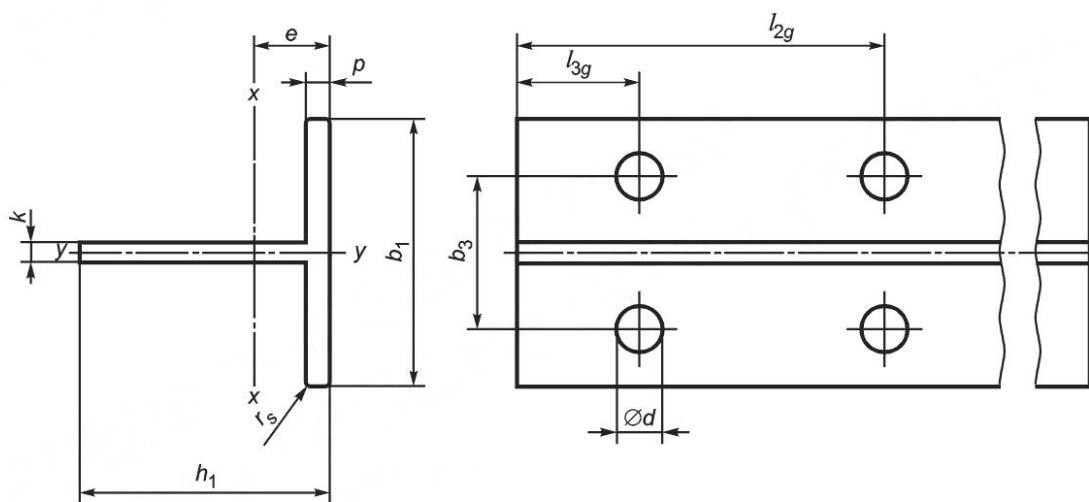
Рисунок 1 — Холоднотянутая направляющая с параллельной кромкой подошвы и головки
