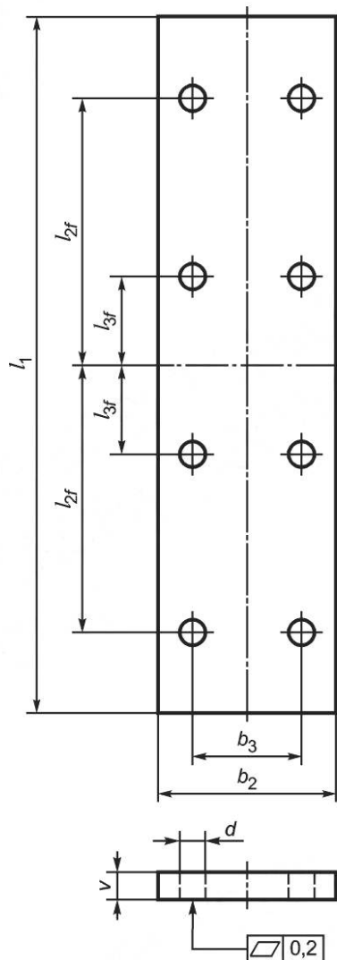
Рисунок 6 — Стыковая планка
