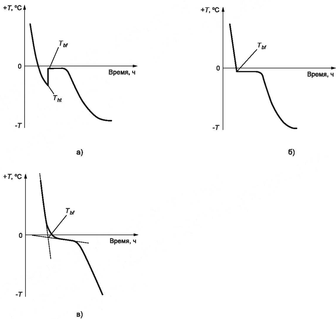
Рисунок Г.1 — Графический метод обработки результатов испытаний по определению температуры начала замерзания T_{bf} [а), б), в)]
