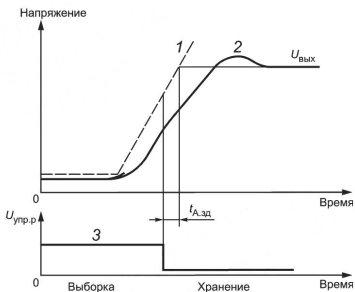
1 — входное напряжение, изменяющееся с заданной скоростью; 2 — выходное напряжение; 3 — диапазон напряжений управления (размах)
