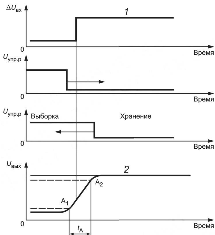
1 — заданный малый перепад входного сигнала; 2 — переходная характеристика; A_1 , A_2 — заданные точки на переходной характеристике
