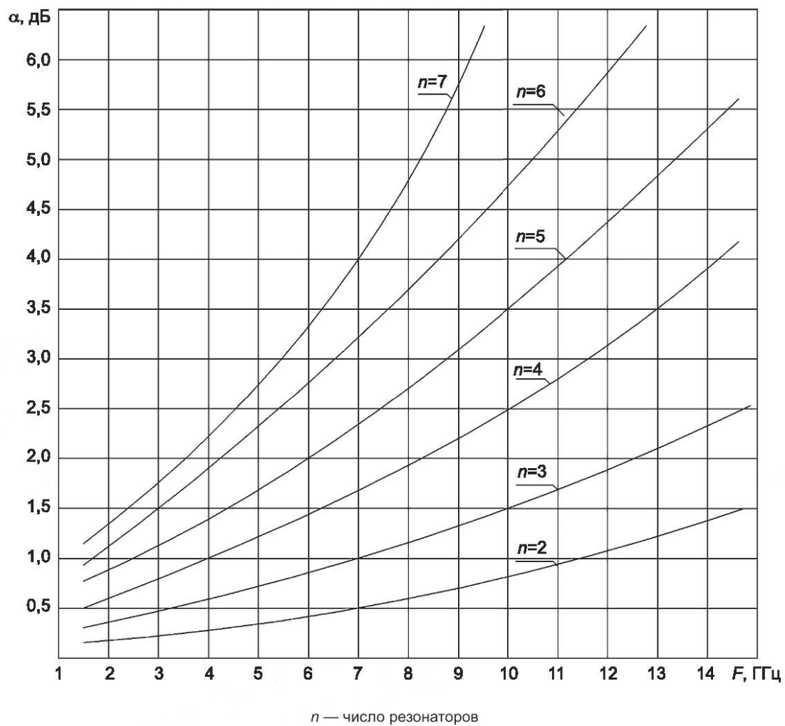
Рисунок 3 — Частотная зависимость минимального затухания \alpha ППФ СВЧ из керамического материала IIIж-4 (КCBH — 1,3)
