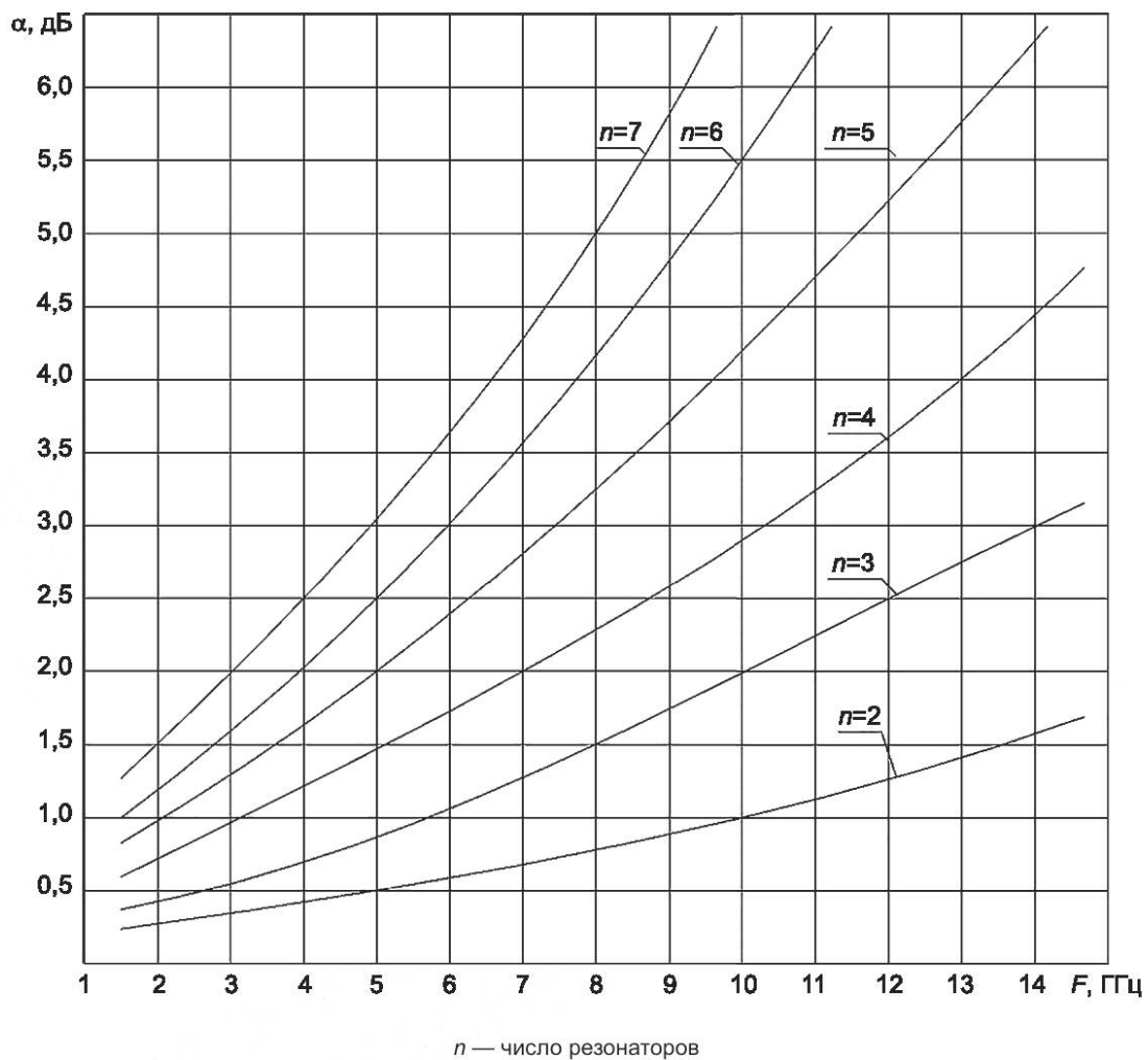
Рисунок 4 — Частотная зависимость минимального затухания \alpha ППФ СВЧ из керамического материала IIIж-4 (КСВН — 1,5)
