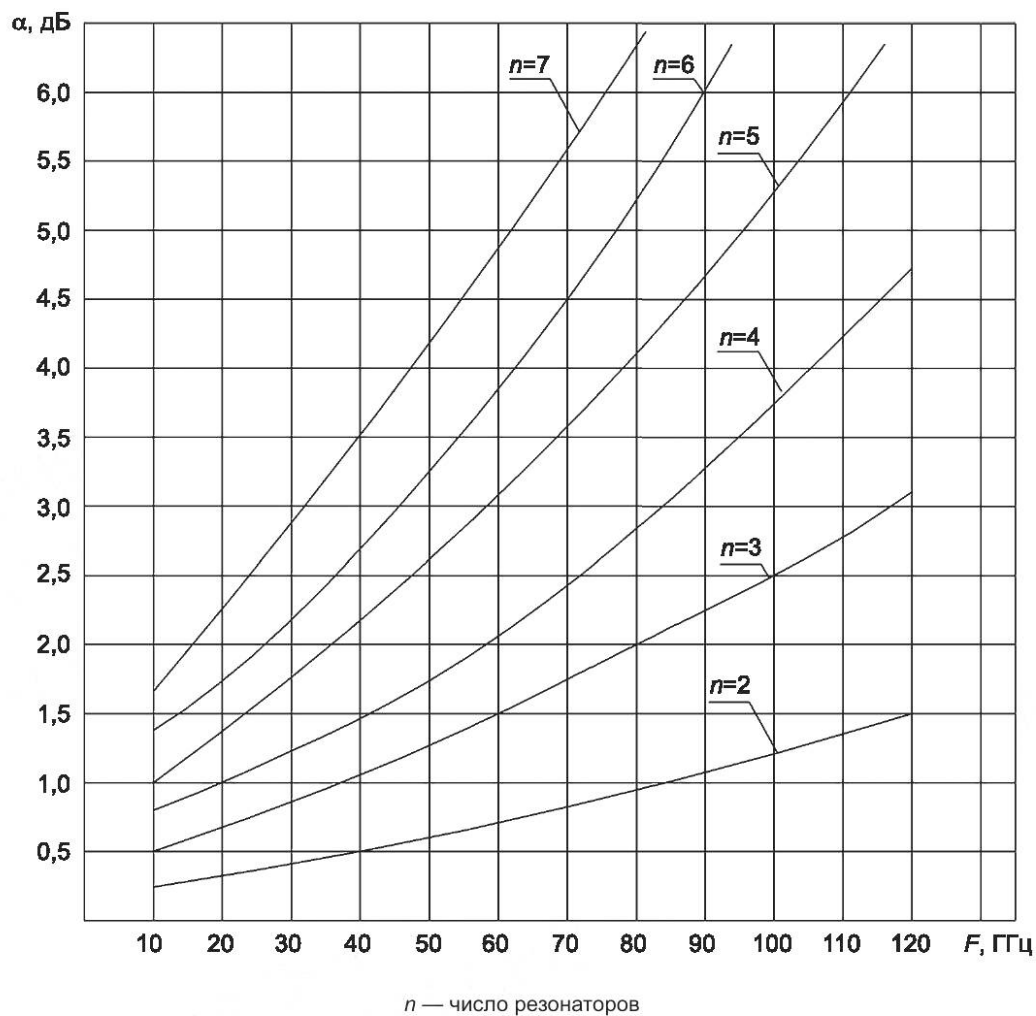
Рисунок 9 — Частотная зависимость минимального затухания \alpha ППФ СВЧ из керамического материала ИИж-4 (КСВН — 1,5)
