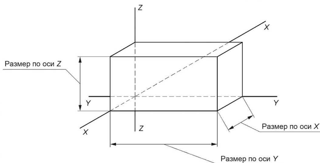
Рисунок 1 — Определение направления осей X , Y , Z в заготовках
