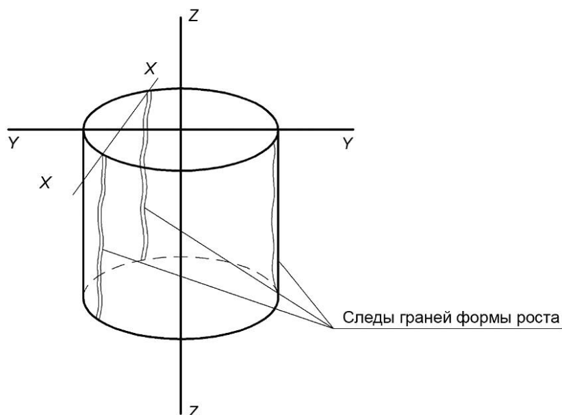
Рисунок 2 — Определение направления осей X , Y исходного кристалла
