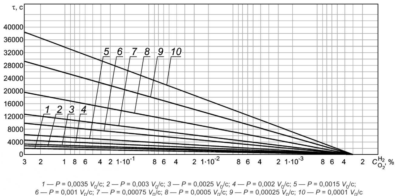
Рисунок В.3 — Ориентировочное время продувки, необходимое для снижения концентрации кислорода от начальной 3,0 \cdot 10^{-4} % при различных расходах газа. Расход газа в долях объема резервуара в с, а суммарный расход в объемах резервуара
