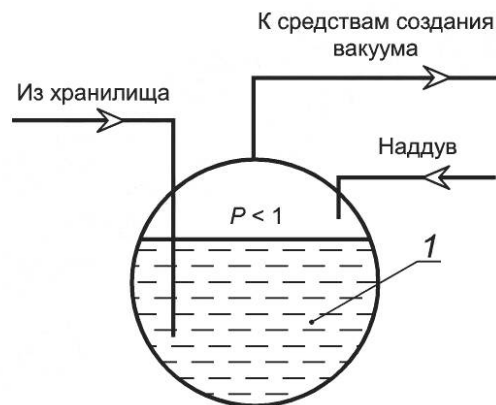
Рисунок Ж.1 — Прямое вакуумирование
