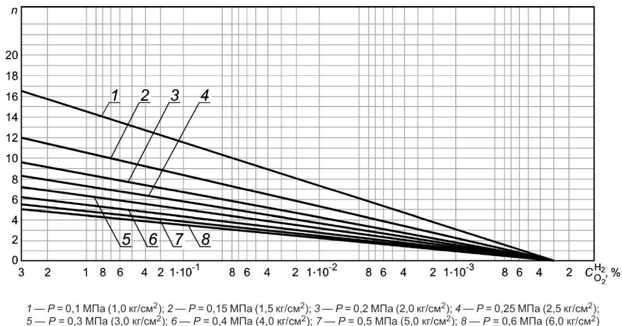
Рисунок В.2 — Ориентировочное число полосканий, необходимое для снижения концентрации кислорода от начальной 3,0 \cdot 10^{-4} \% при различных давлениях наддува (давление при сбросе газа очистки 0,015 МПа ( 0,015 кгс/см 2 ))
