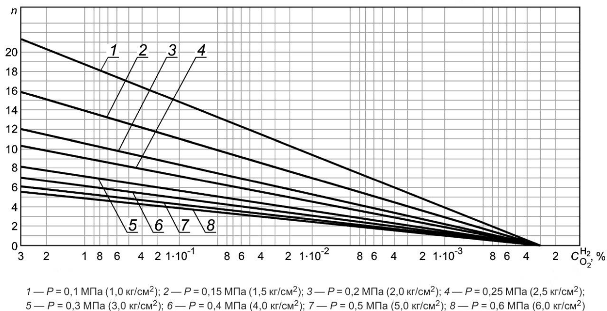
Рисунок В.1 — Ориентировочное число полосканий, необходимое для снижения концентрации кислорода от начальной 3,0 \cdot 10^{-4} \% при различных давлениях наддува (давление при сбросе газа очистки 0,03 МПа ( 0,3 кг/см 2 ))
