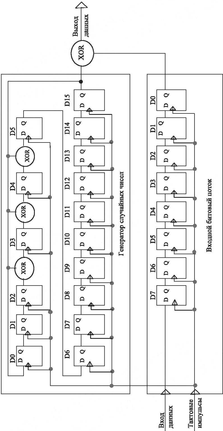
Рисунок 10.2 — Скремблер/дескремблер
