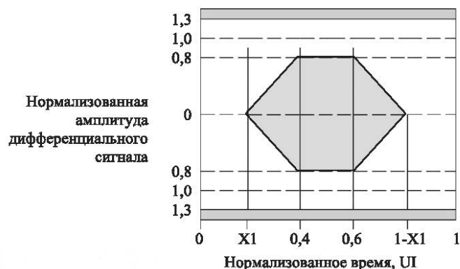
Рисунок 7.13 — Электрооптическая маска глазковой диаграммы передатчиков, предназначенных для работы в диапазоне битовых скоростей от 1 до 5 Гбит/с
