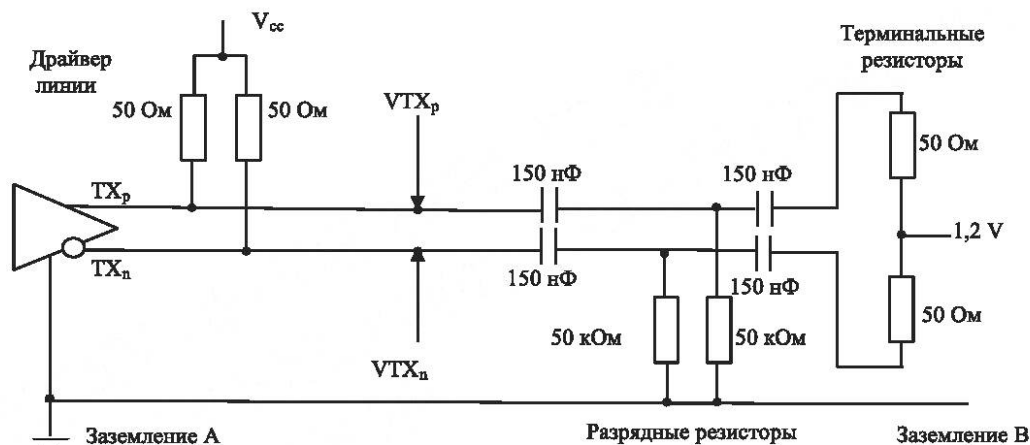
Рисунок 7.3 — Сигналы последовательного выхода
