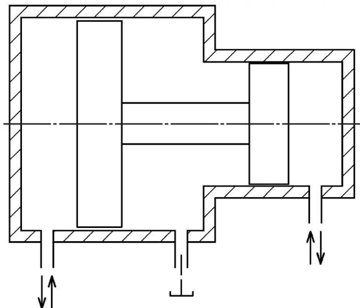
Рисунок 25 — Поступательный гидропреобразователь
