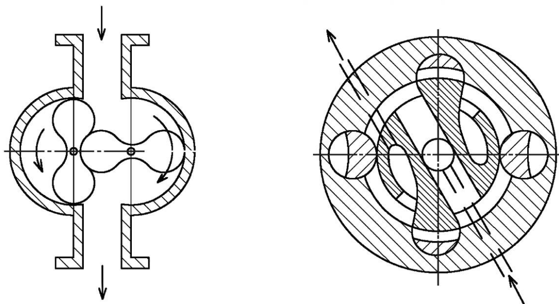
Рисунок 14 — Коловратный гидромотор
