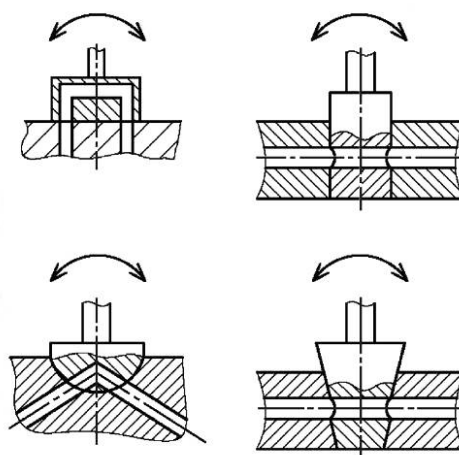
Рисунок 28 — Крановый гидроаппарат
