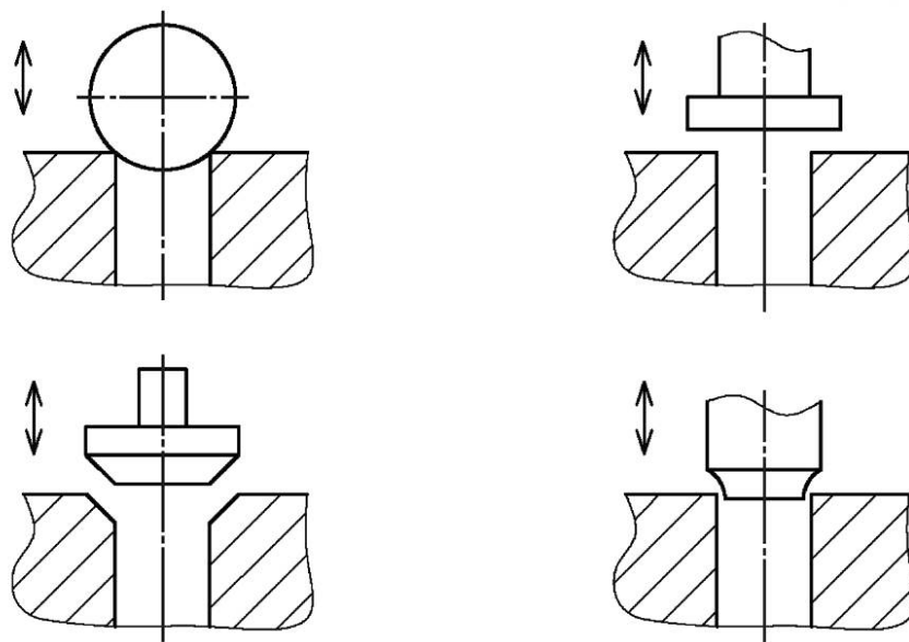
Рисунок 29 — Клапанный гидроаппарат
