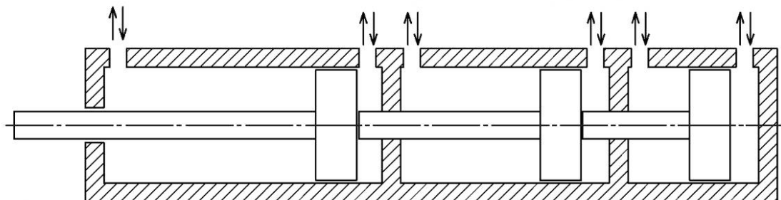
Рисунок 4 — Многопозиционный гидроцилиндр
