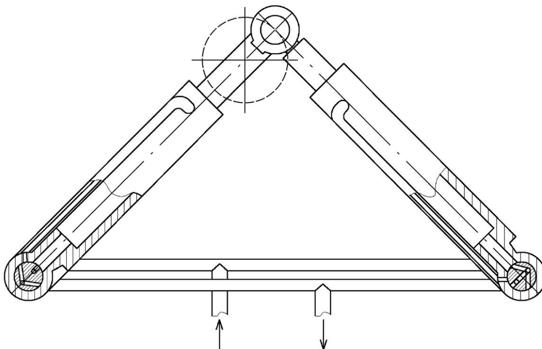
Рисунок 22 — Кривошипный гидромотор
