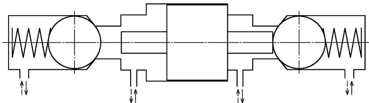
Рисунок 45 — Двухсторонний гидрозамок
