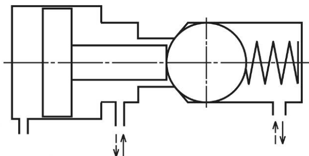
Рисунок 44 — Односторонний гидрозамок
