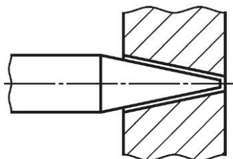
Рисунок 37 — Гидродроссель
