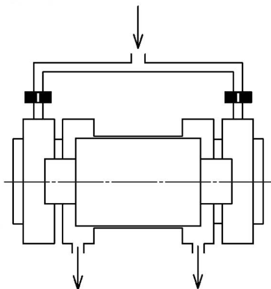
Рисунок 39 — Дресселирующий синхронизатор расходов
