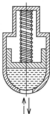
Рисунок 49 — Пружинный гидроаккумулятор
