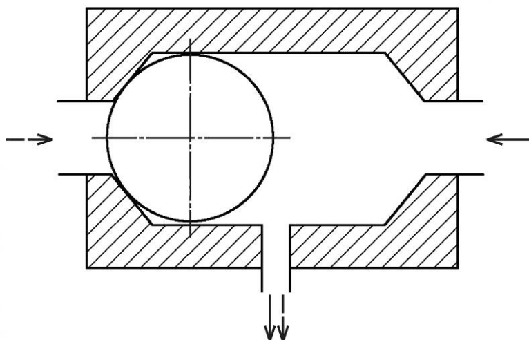
Рисунок 47 — Гидроклапан «ИЛИ»
