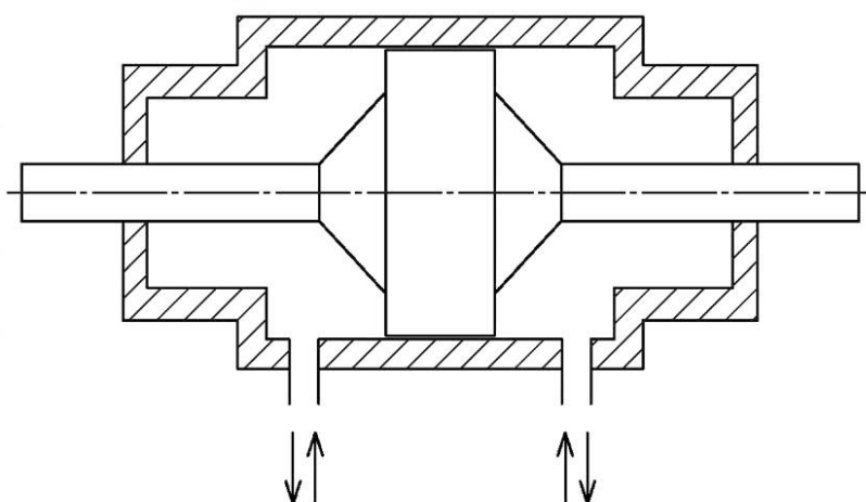
Рисунок 10 — Гидроцилиндр с торможением
