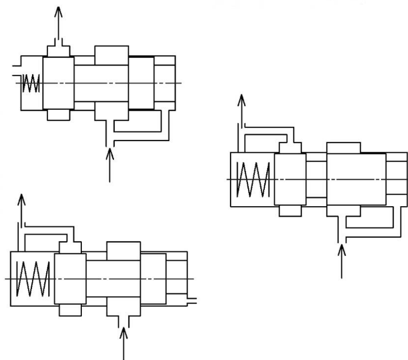
Рисунок 34 — Регулятор разности давлений
