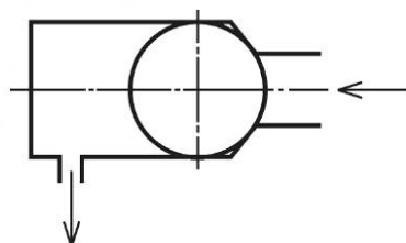
Рисунок 43 — Обратный гидроклапан
