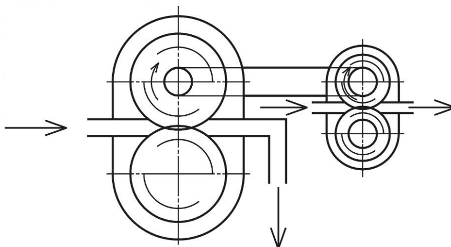
Рисунок 26 — Вращательный гидропреобразователь
