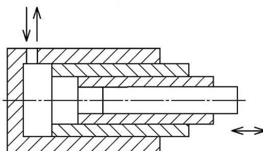
Рисунок 9 — Телескопический гидроцилиндр
