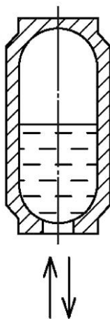
Рисунок 51 — Пневмогидроаккумулятор
