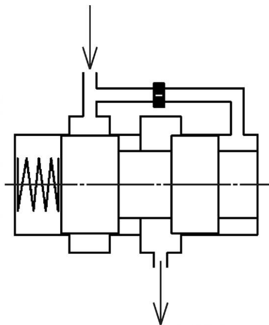
Рисунок 42 — Гидроклапан последовательности
