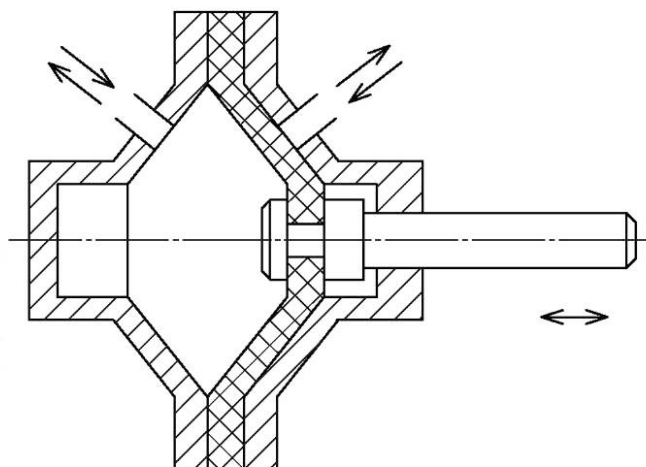
Рисунок 7 — Мембранный гидроцилиндр
