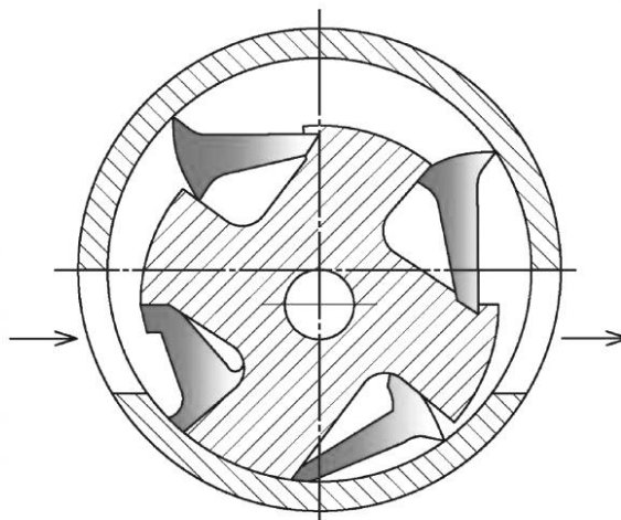
Рисунок 19 — Фигурно-шиберный гидромотор
