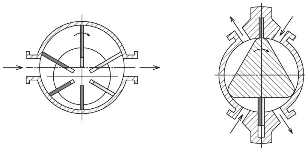
Рисунок 18 — Пластинчатый гидромотор
