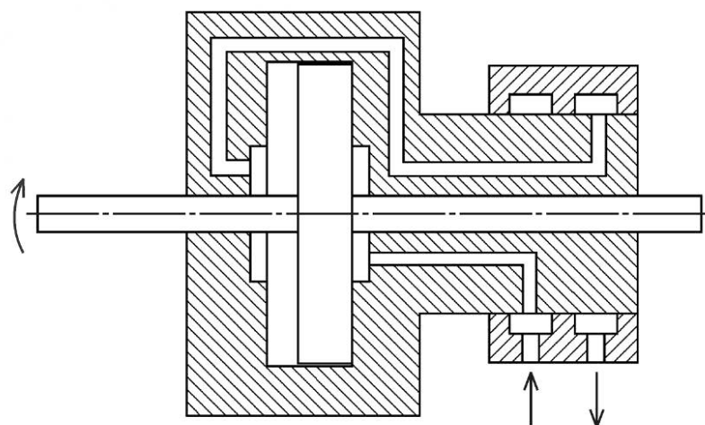
Рисунок 54 — Вращающийся гидроцилиндр
