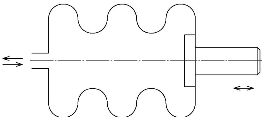
Рисунок 8 — Сильфонный гидроцилиндр
