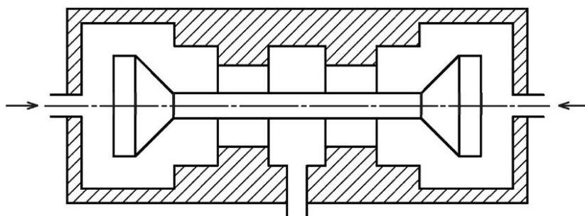
Рисунок 46 — Гидроклапан «И»
