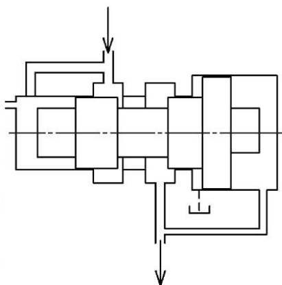
Рисунок 36 — Предохранительный гидроклапан
