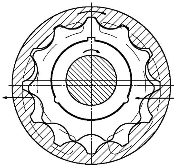
Рисунок 17 — Героторный гидромотор
