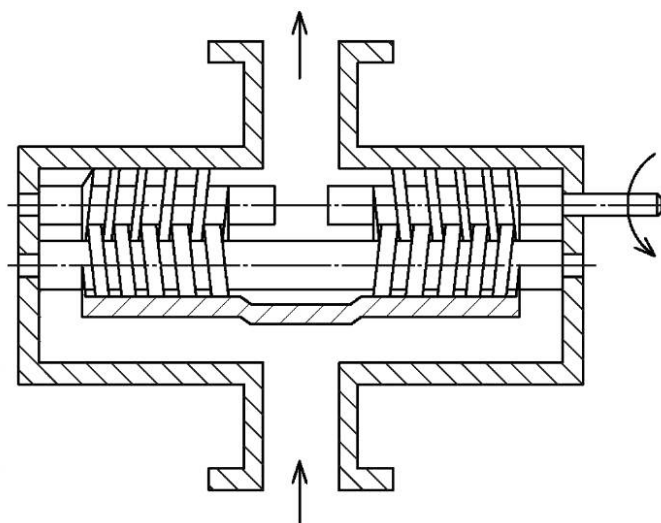
Рисунок 15 — Винтовой гидромотор
