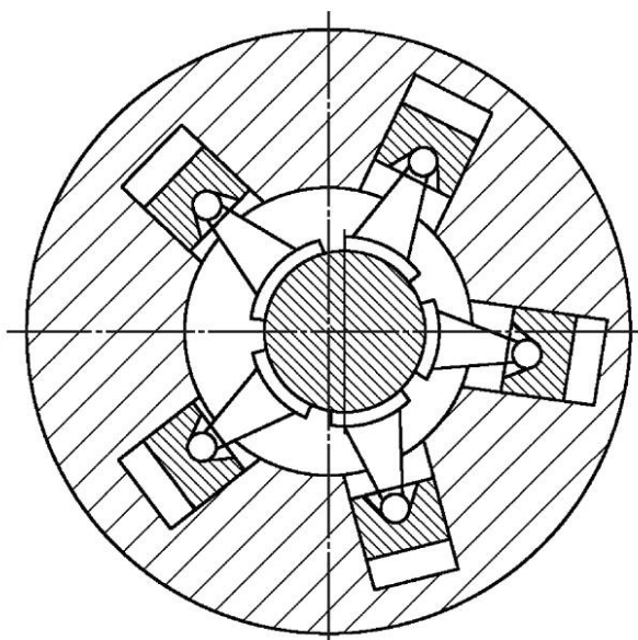
Рисунок 24 — Гидромотор с внутренним кулачком
