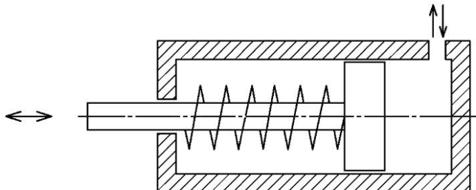
Рисунок 2 — Гидроцилиндр одностороннего действия
