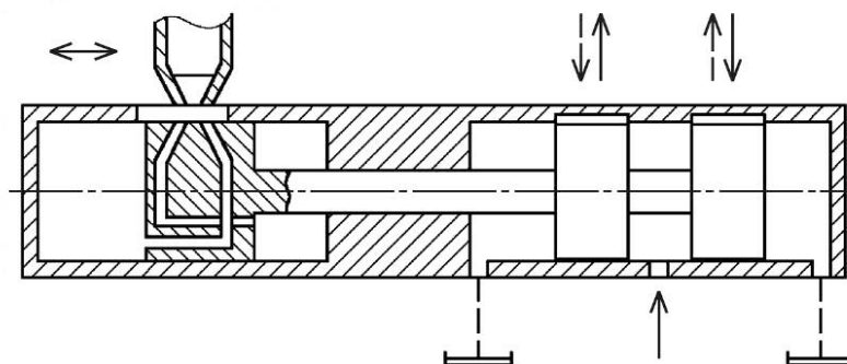
Рисунок 53 — Гидроусилитель
