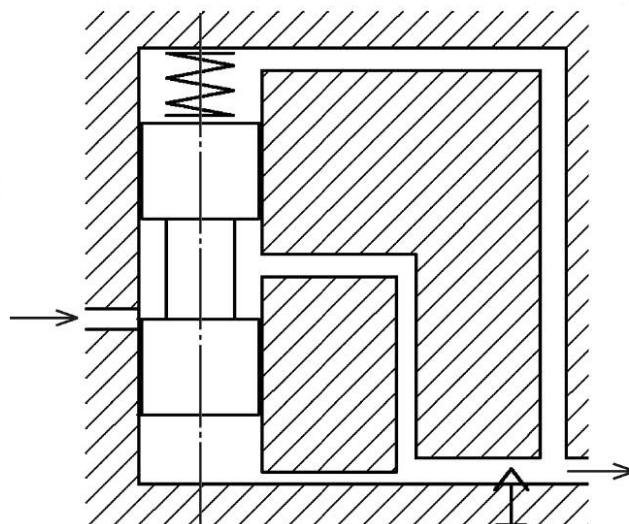
Рисунок 38 — Регулятор расхода
