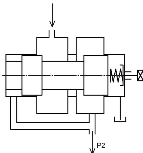
Рисунок 33 — Редуциционный регулятор давления
