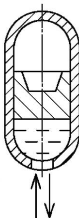
Рисунок 52 — Поршневой пневмогидроаккумулятор
