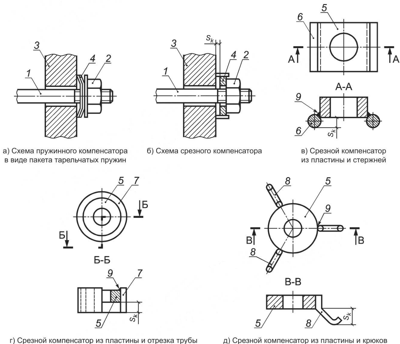
Рисунок 5 — Конструкции компенсаторов в узлах соединения с анкерной плитой или с лицевым элементом
