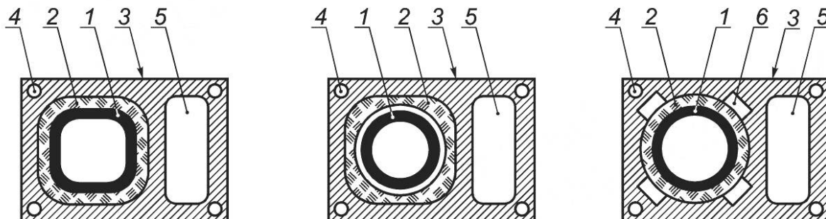
1 — внутренняя оболочка; 2 — теплоизоляция или воздушный зазор; 3 — наружная оболочка; 4 — отверстия для креплений; 5 — шахта подачи воздуха для горения; 6 — каналы проветривания
