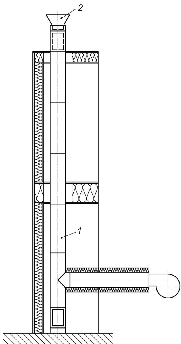
Рисунок 2 — Испытание конструкции для удаления дымовых газов на истирание
