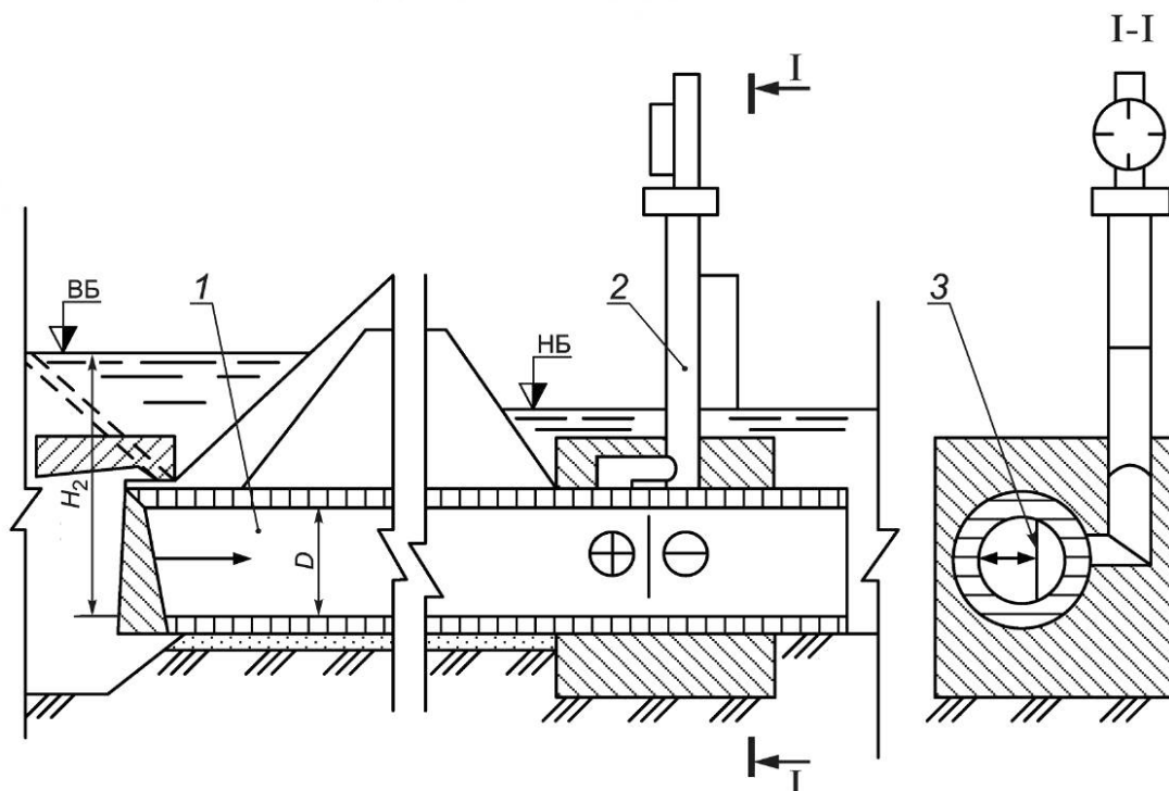
Рисунок Д.7 — Схема трубчатого расходомера-регулятора с насадком на входе
