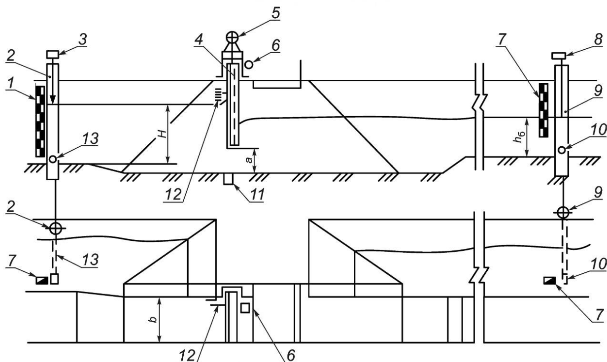
1, 7 — контрольные рейки; 2, 9 — колодцы; 3, 8 — измерительные преобразователи напора; 4 — сооружение с затвором; 5 — подъемный механизм затвора; 6 — измеритель высоты открытия затвора; 10, 13 — импульсные трубки; 11 — импульсное уплотнение; 12 — указатель высоты затвора; H — глубина воды в верхнем бьефе, м; h_6 — глубина воды в нижнем бьефе, м; a — высота выходного сечения, м; b — ширина канала по дну, м
