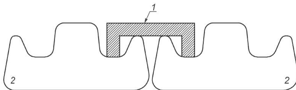
в) Т-образный 1 (армирующий профиль, обеспечивающий стойкость к давлению)
