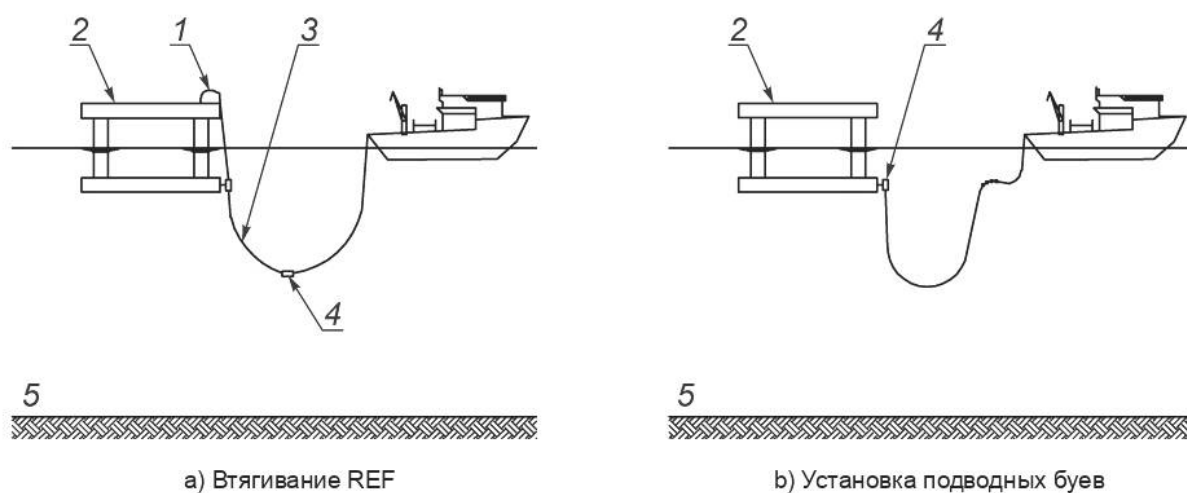
Рисунок 34 — Типовая процедура установки райзера в конфигурации крутого S-подъема
