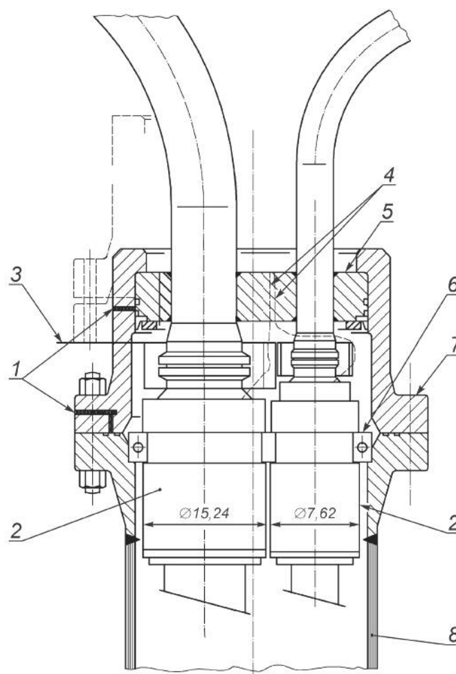
Рисунок 16 — Пример типовой конструкции основания райзера
