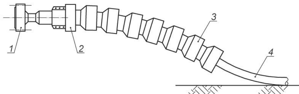
а) Ограничители изгиба, покрывающие гибкую трубу
