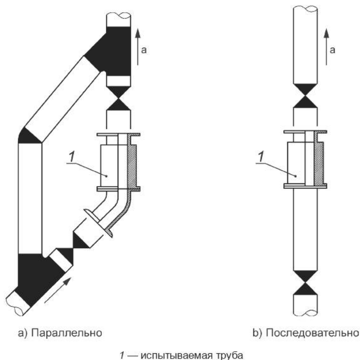
Рисунок 38 — Схема возможного расположения испытываемой трубы
