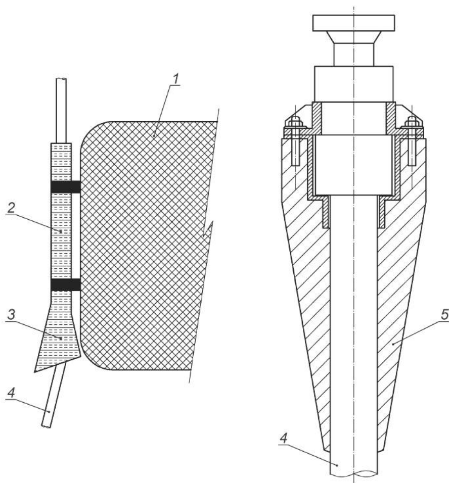
1 — понтон; 2 — I-образная труба; 3 — раструб; 4 — гибкий райзер; 5 — элемент жесткости на изгиб
