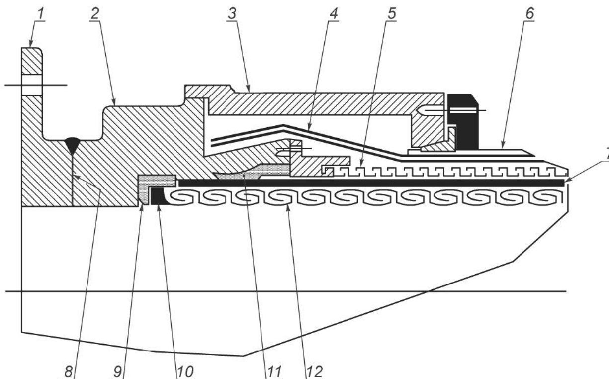
1 — монтажный фланец; 2 — корпус концевой фитинга (внутренняя оболочка); 3 — корпус концевой фитинга (наружная оболочка); 4 — армирующий слой, работающий на растяжение (залитый эпоксидным материалом); 5 — армирующий слой, обеспечивающий стойкость к давлению; 6 — наружная оболочка; 7 — внутренняя оболочка, работающая под давлением (и защитные слои); 8 — шейка концевой фитинга; 9 — торцевое уплотнение; 10 — замыкающее кольцо каркаса; 11 — радиальное уплотнение; 12 — каркас
