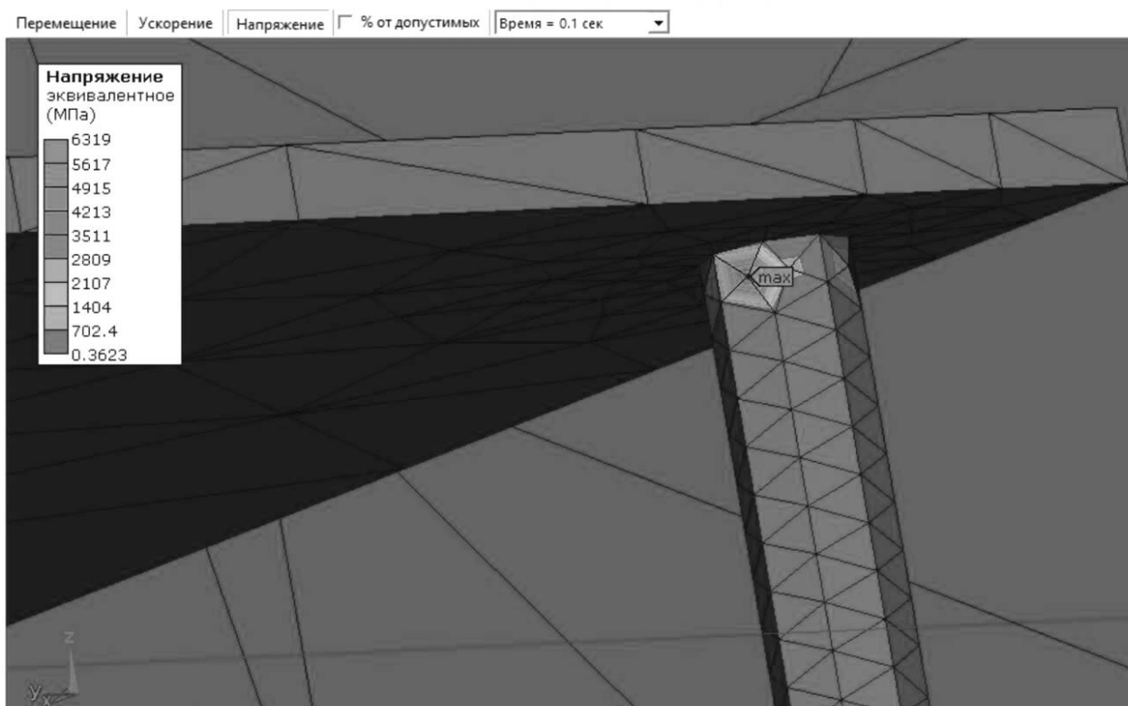
Рисунок А.8 — Эквивалентные механические напряжения во всех точках конструкции блока ЭА при воздействии линейного ускорения в заданный момент времени
