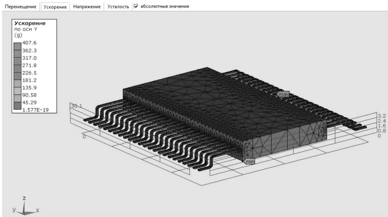
Рисунок А.7 — Среднеквадратические ускорения по оси Y во всех точках конструкции ЭКБ
