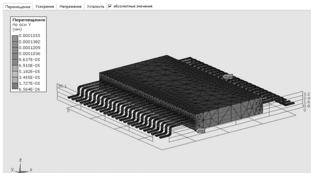
Рисунок А.6 — Среднеквадратические перемещения по оси Y во всех точках конструкции ЭКБ
