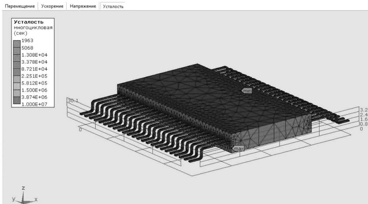
Рисунок А.9 — Время до усталостного разрушения во всех точках конструкции ЭКБ при воздействии случайной вибрации
