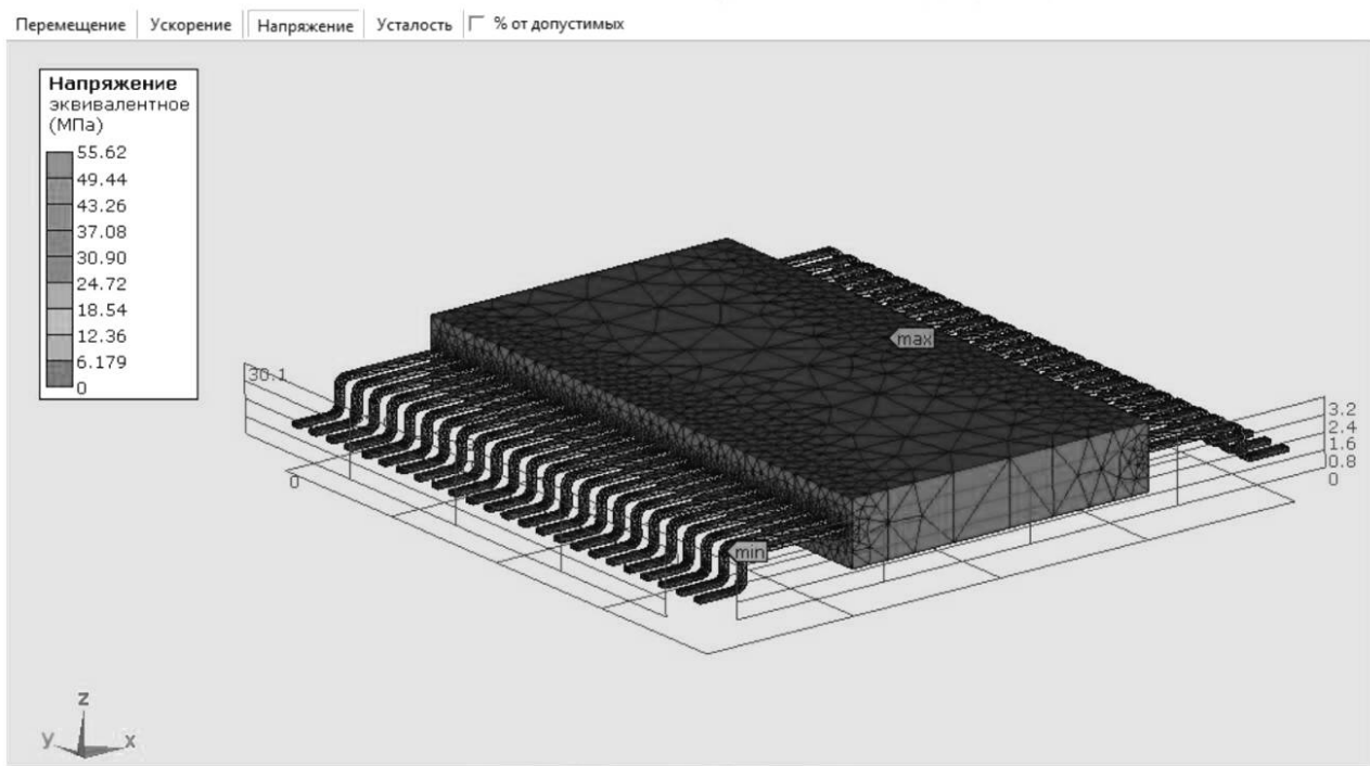
Рисунок А.8 — Среднеквадратические эквивалентные механические напряжения во всех точках конструкции ЭКБ
