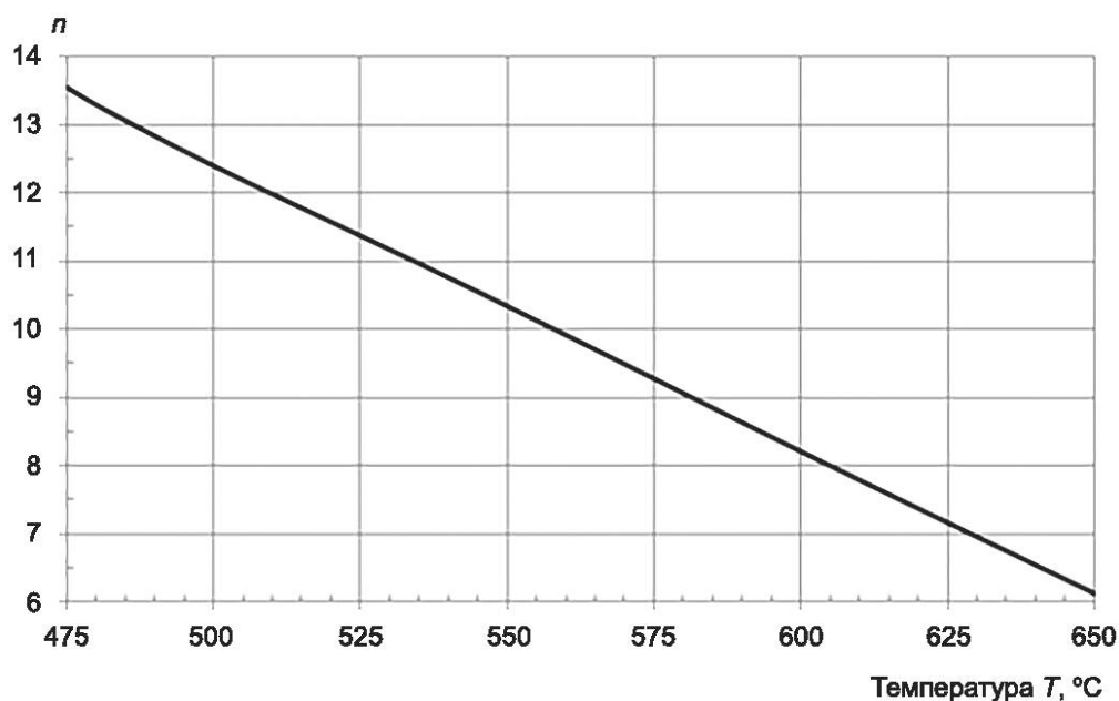
Рисунок Б.9 — График определения показателя степени в уравнении длительной прочности для стали марки 10Х9МФБ
