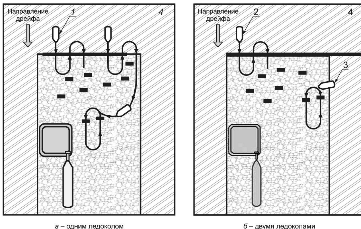
Рисунок Е.1 — Схема разрушения протяженных торосистых образований (гряд торосов)
