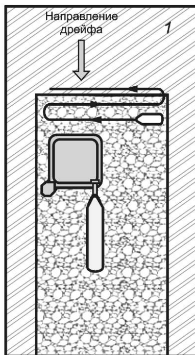
Рисунок Д.2 — Схема разрушения ледяных полей при применении линейного метода 2
