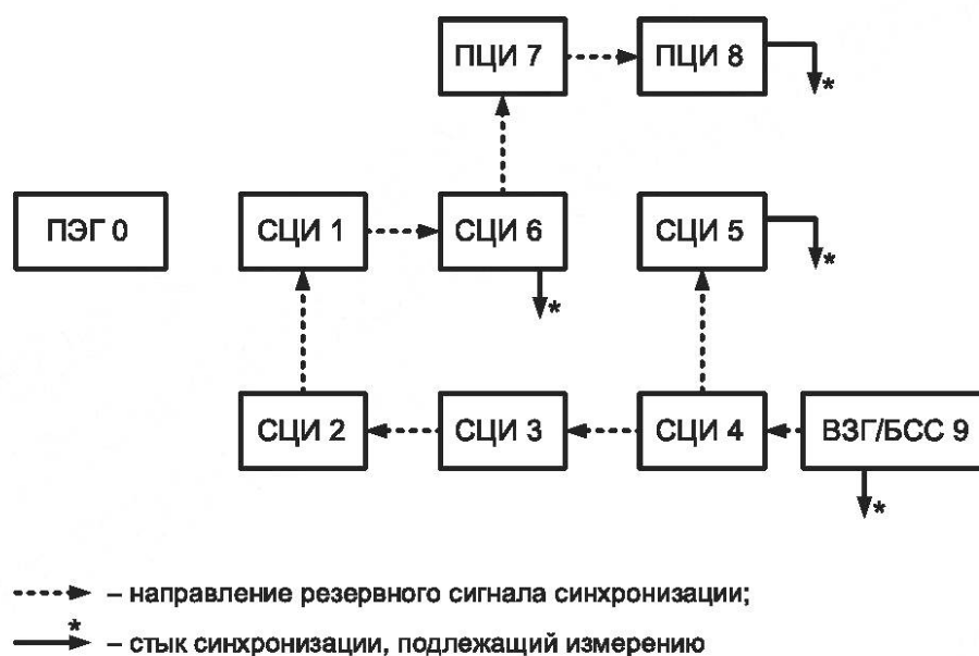
Рисунок А.3 — Граф прохождения резервного сигнала синхронизации
