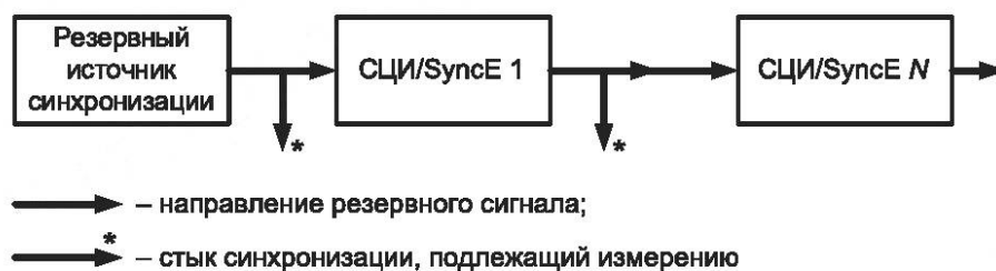
Рисунок 4 — Схема измерений параметров синхронизации по пункту 4 таблицы 1
