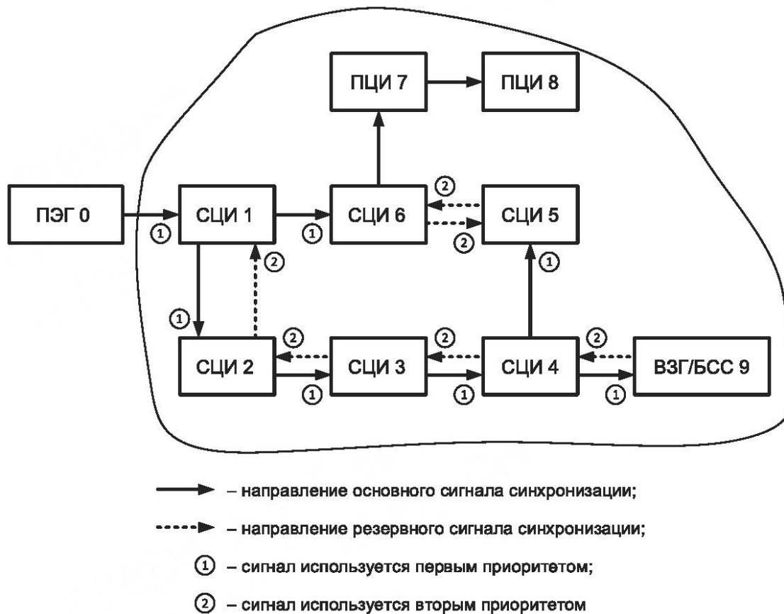
Рисунок А.1 — Пример схемы участка сети ТСС
