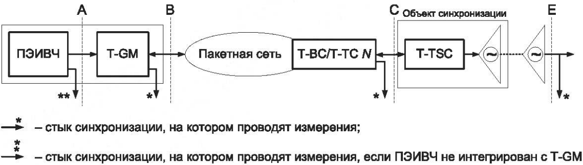
Рисунок 12 — Стыки синхронизации сети СШВ, подлежащие измерению, когда T-TSC встроен в объект синхронизации
