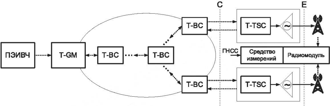
Рисунок 18 — Вариант измерения максимальной относительной ошибки времени в полевых условиях на основе измерения параметров радиосигналов
