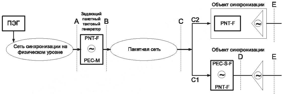
Рисунок 14 — Контрольные точки сети синхронизации частоты на основе пакетных технологий [телекоммуникационный профиль PTP (см. [11])]
