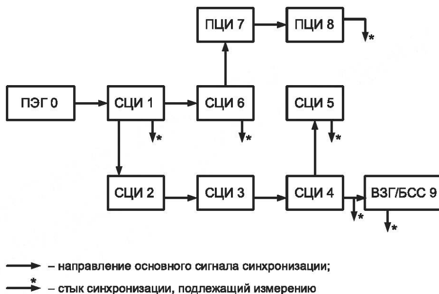
Рисунок А.2 — Граф прохождения основного сигнала синхронизации
