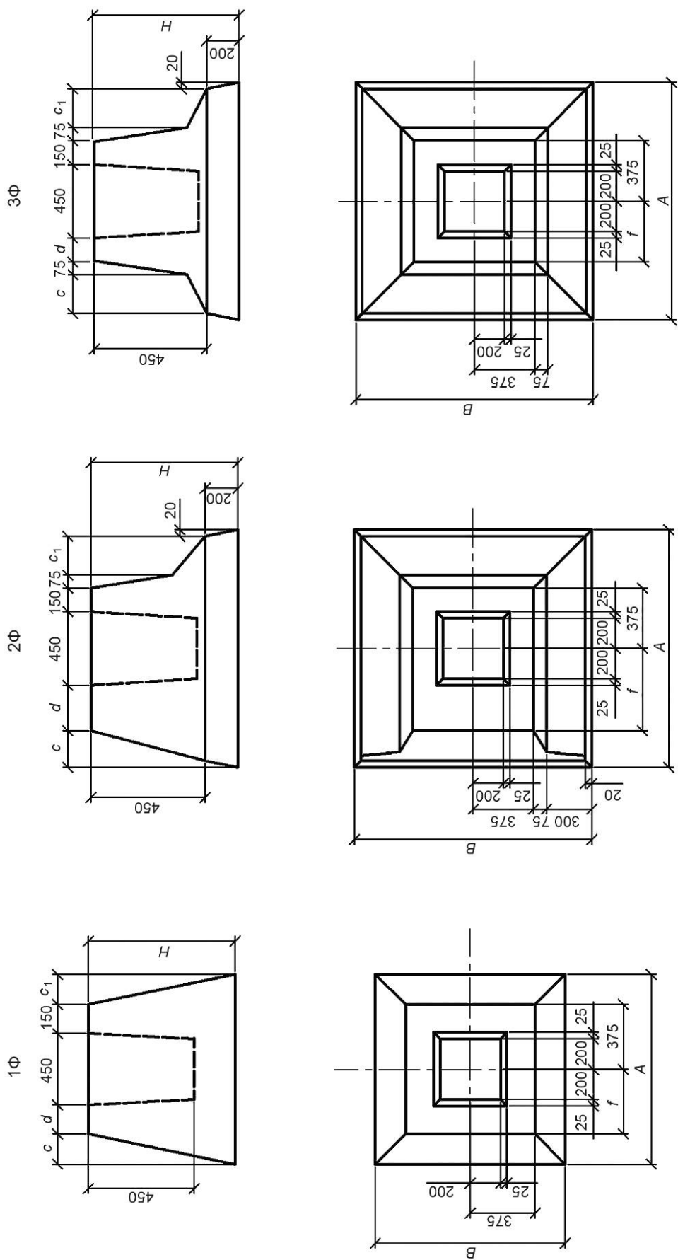
Рисунок 1 — Фундаменты сельскохозяйственных зданий
