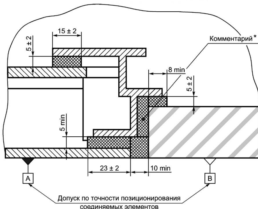
Рисунок Г.5 — Пример указания размеров клеевых соединений
