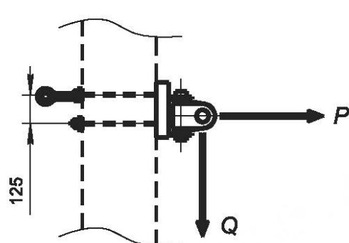
а) узел крепления тяги консоли на закладных деталях
