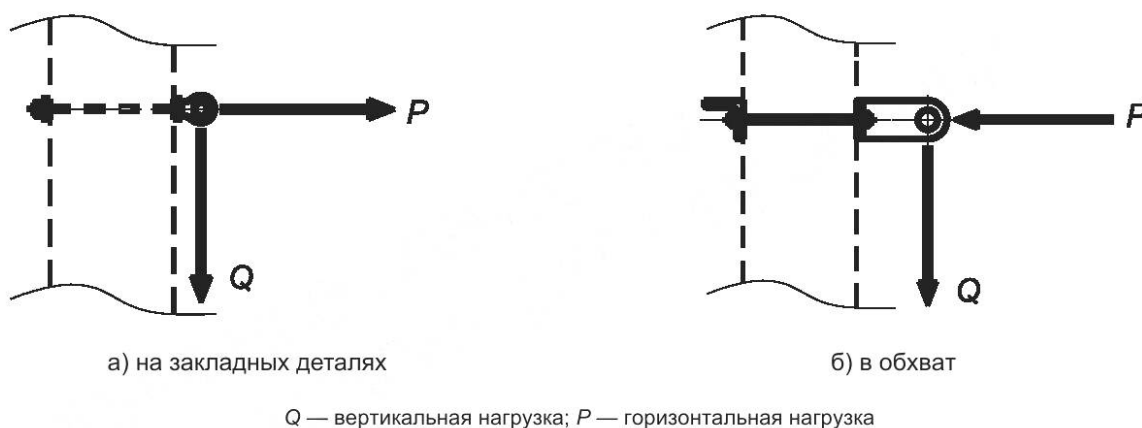
Рисунок 45 — Схемы приложения нагрузок к узлам крепления кронштейна
