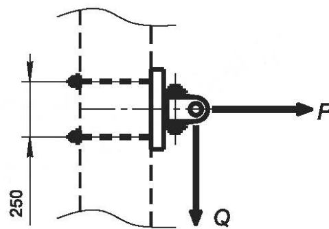
б) узел крепления пяты консоли на закладных деталях
