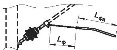
а) основные размеры
