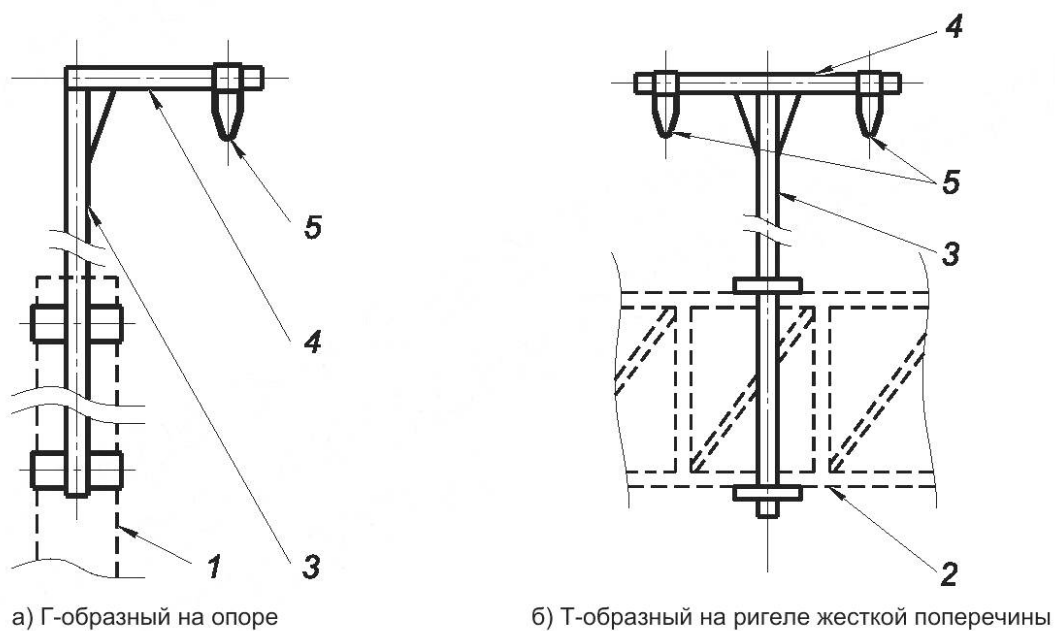
Рисунок 9 — Элементы конструкции основных видов кронштейнов с вертикальной стойкой, предназначенных для крепления проводов питающих линий, питающих, усиливающих и/или экранирующих проводов
