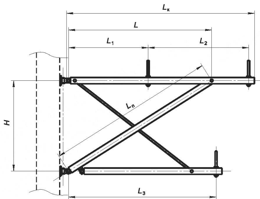
а) основные размеры
