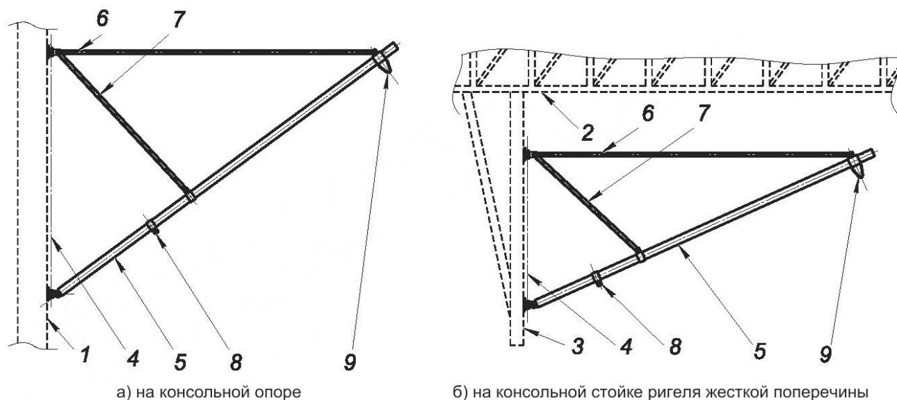
Рисунок 1 — Элементы конструкции однопутной наклонной консоли
