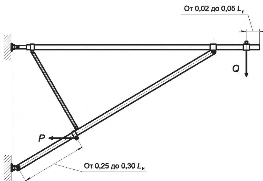
б) схема приложения нагрузок
