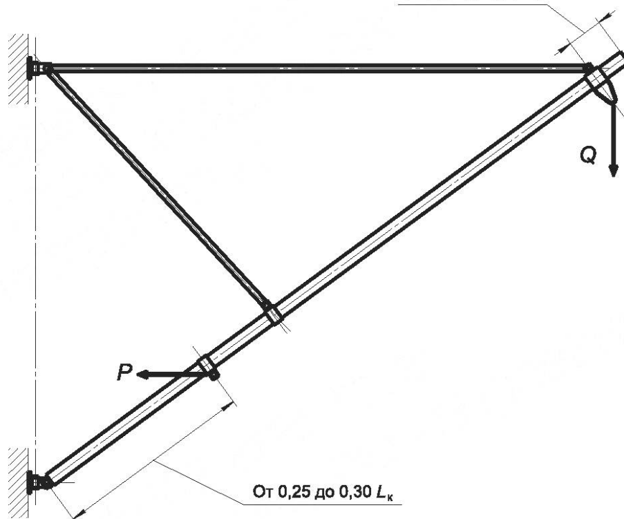
б) схема приложения нагрузок
