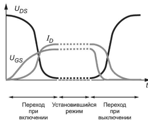
г) Коммутация резистивной нагрузки
