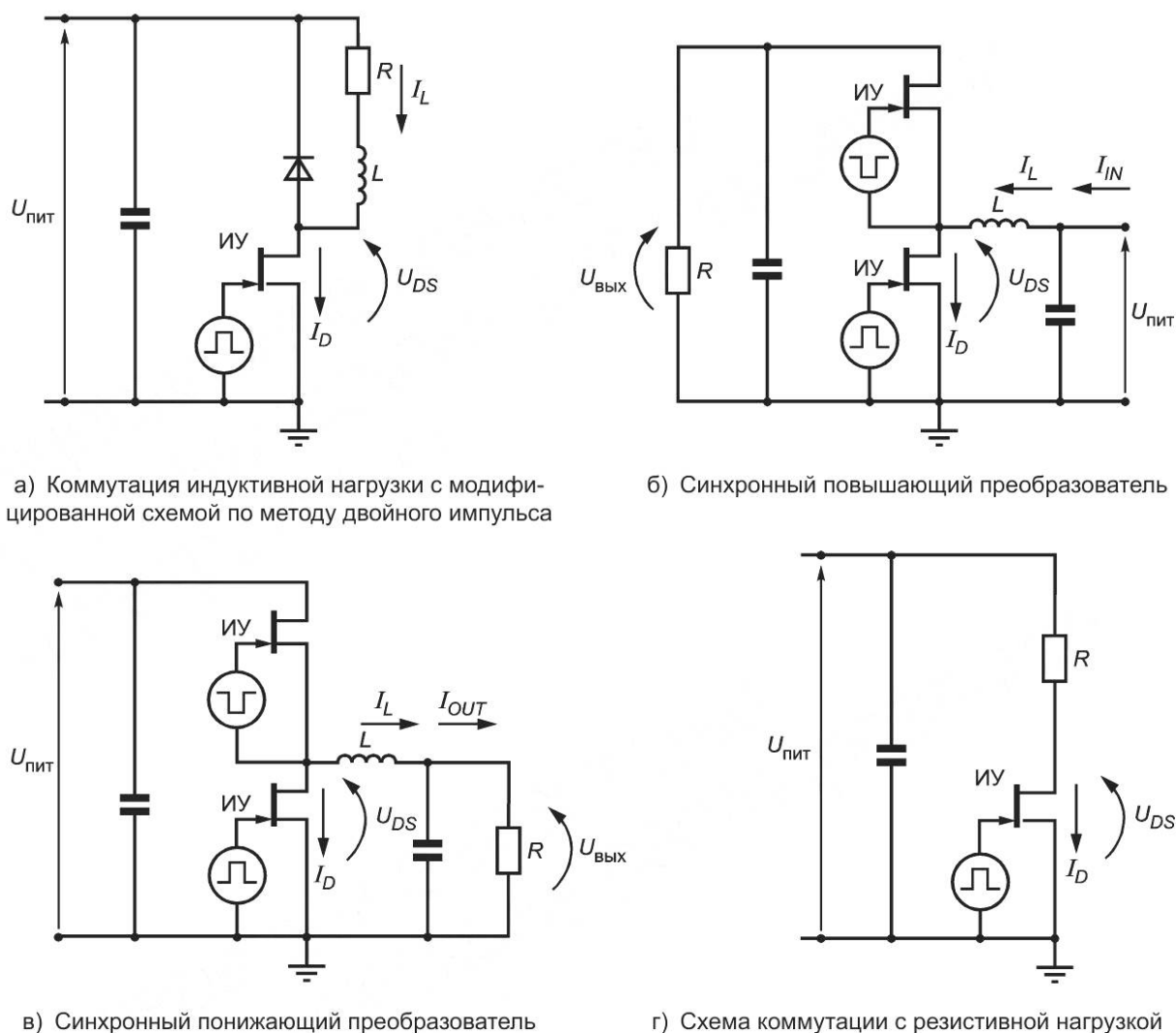
Рисунок 2 — Примеры схем, обеспечивающих режим непрерывной коммутации с настраиваемой областью I_D — U_{DS}
