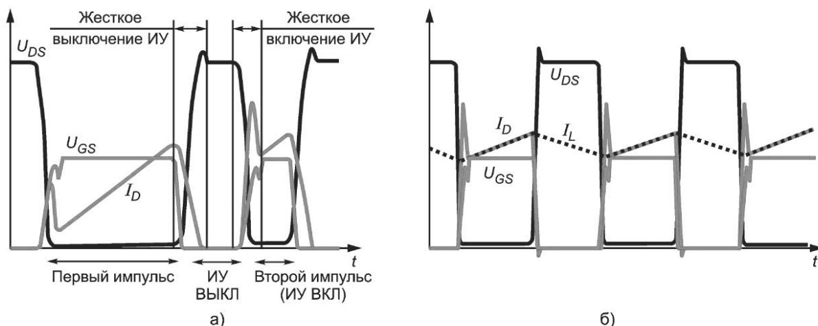
Рисунок 3 — Формы U_{GS} , U_{DS} и I_D
