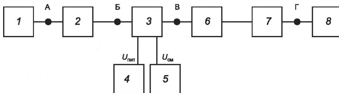
1 — СВЧ-генератор; 2 — изолятор; 3 — ИУ; 4 — источник питания; 5 — источник напряжения смещения; 6 — аттенюатор; 7 — полосно-пропускающий фильтр; 8 — измеритель мощности; U_{пит} и U_{см} — напряжения питания и смещения соответственно
