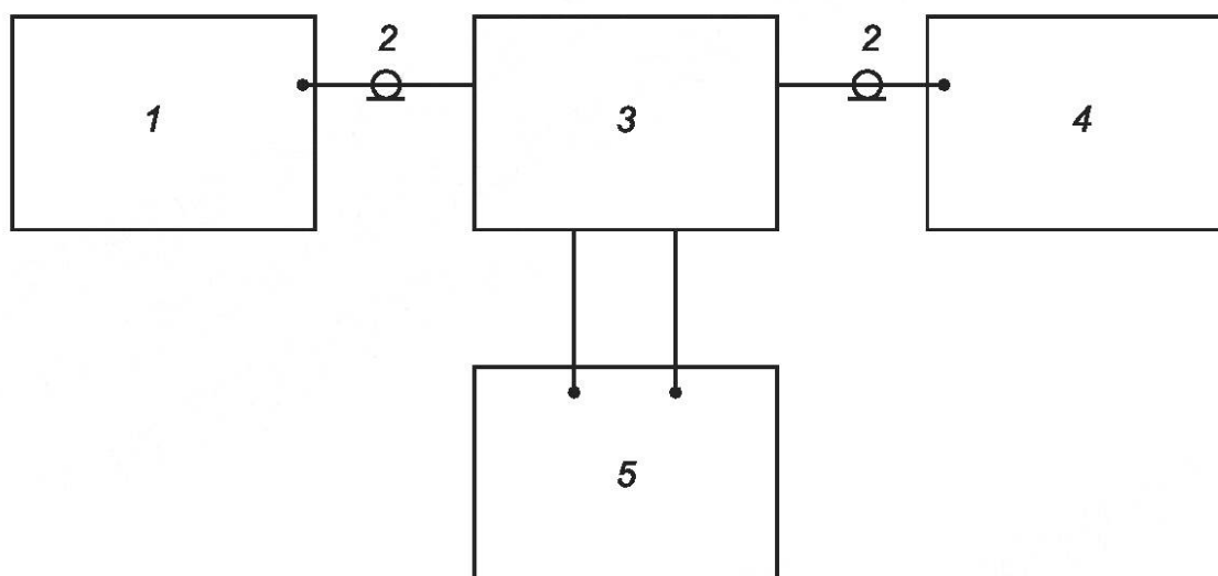
Рисунок 11 — Схема измерений рабочего диапазона частот ИУ
