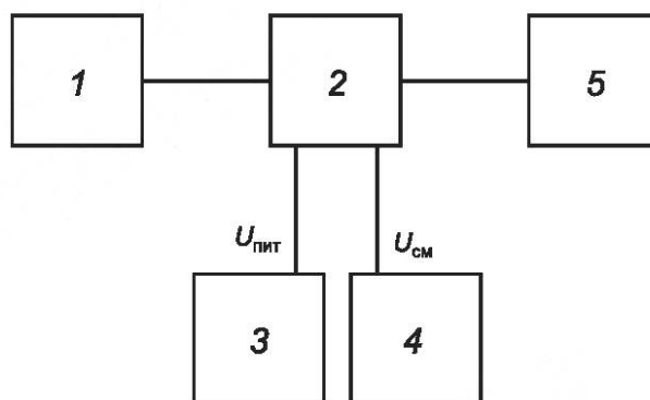
1 — рефлектометр; 2 — ИУ; 3 — источник питания; 4 — источник напряжения смещения; 5 — согласованная нагрузка
