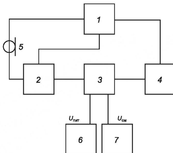
1 — САЦ; 2 — датчик КСВН; 3 — ИУ; 4 — детекторная головка; 5 — СВЧ кабельная сборка; 6 — источник питания; 7 — источник напряжения смещения; U_{\text{ПИТ}} и U_{\text{СМ}} — напряжения питания и смещения соответственно
