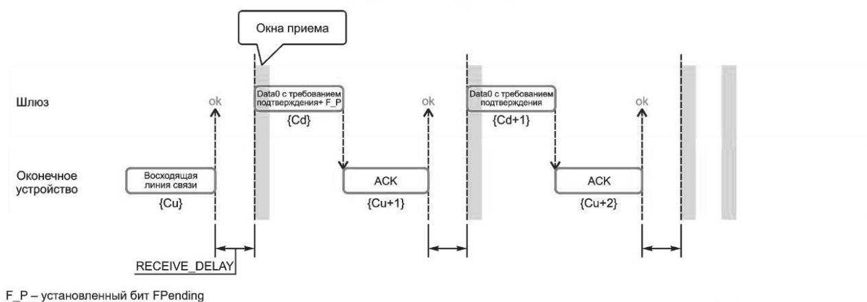
Рисунок 65 — Диаграмма передачи очереди нисходящих сообщений (пример 1)
