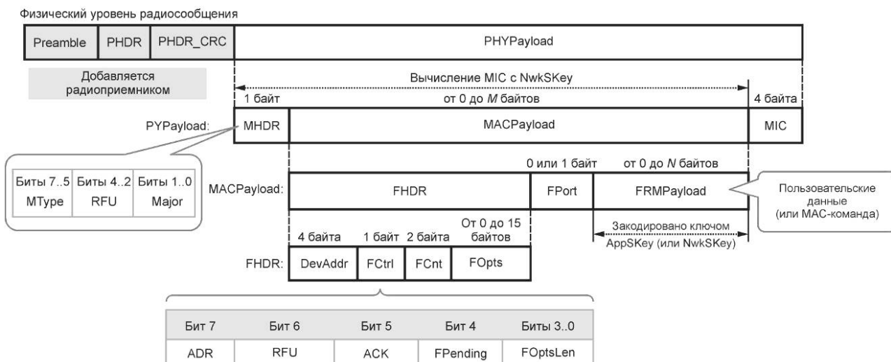
Рисунок 4 — Структура нисходящего радиосообщения на физическом уровне
