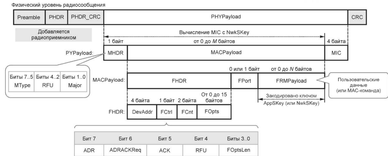
Рисунок 3 — Структура восходящего радиосообщения на физическом уровне
