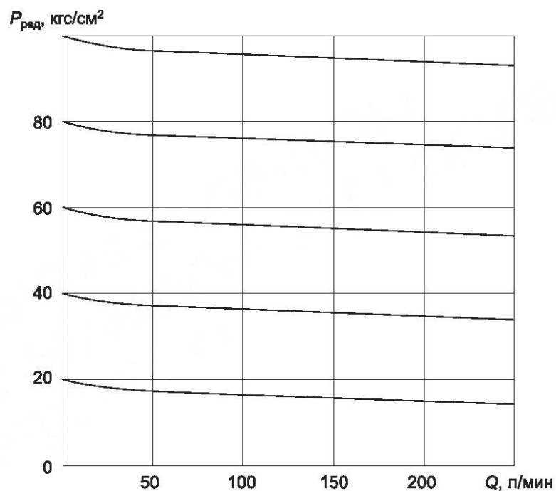
Рисунок А.14 — Типовая форма диаграммы изменения редуцированного давления при изменении расхода при различных значениях редуцированного давления p_{\text{ред}} = f(Q)
