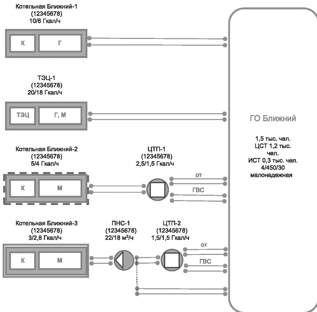
Схема системы теплоснабжения с атрибутами элементов
